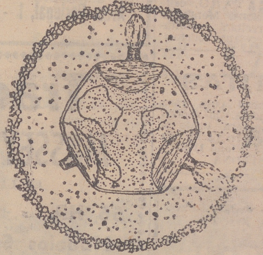
Dibujo de unos «elementos organizados» observados por Claus y Nagy en meteoritos (de la revista «Nature»)
