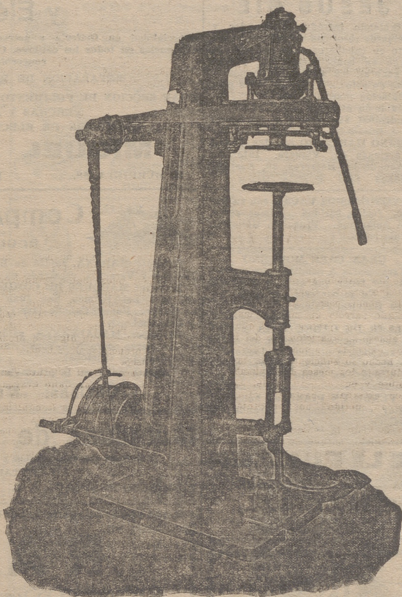
Máquina cerradora a lata parada, capaz para cierres hasta 500 milímetros de diámetro y lata petrolera.
