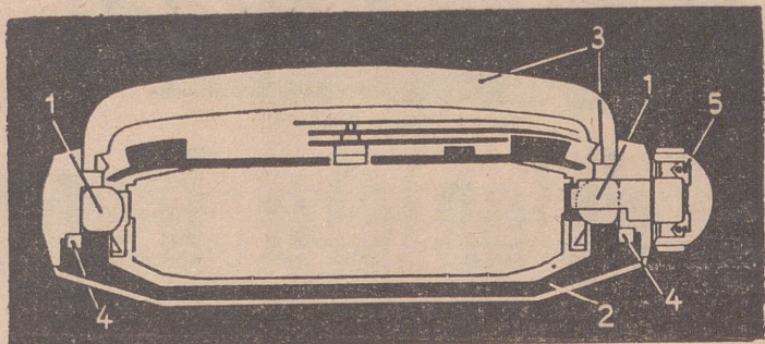
1.- JUNTA ELASTICA. 3.- CRISTAL ARMADO. 2.- FONDO DE ACERO ROSCADO. 4 y 5.- JUNTAS IMPERMEABLES.
