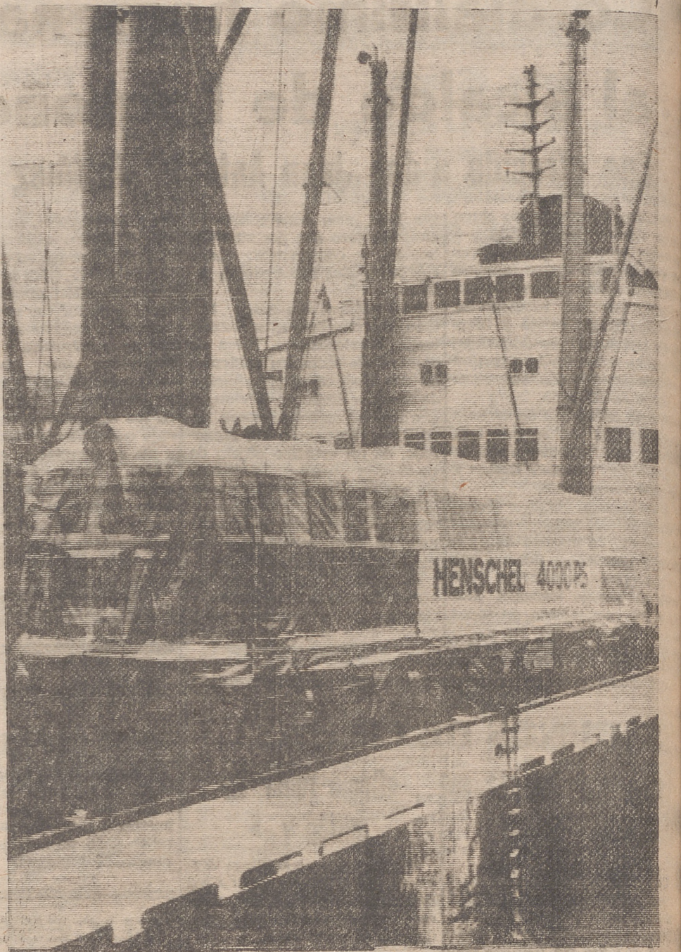
Una locomotora Diesel-Henschel, de 4.000 H.P., que tiene 23 metros de longitud, metro de altura y un peso de 130 toneladas, ha sido embarcada en el puerto de la ciudad alemana de Hamburgo para su transporte de Tsingtao (China continental). Tardará en ca de dos meses en recorrer las 11.000 millas de distancia. La locomotora podrá alcanzar una velocidad media de 160 kilómetros por hora. — (Foto Afp).
