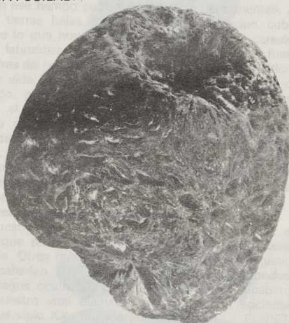
ESPONJA FOSILIZADA. DEHESA DE NAVARRETE 600 Millones de años
