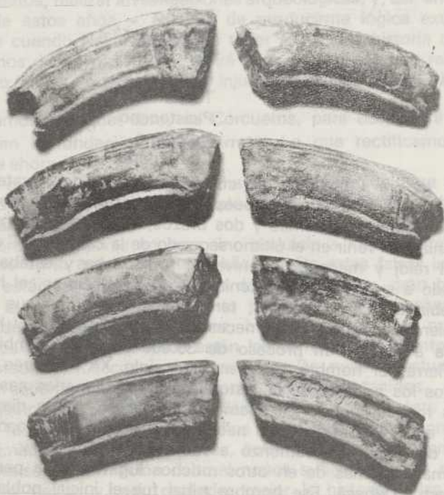
MOLARES DEL ELEFANTE PRIMITIVO (MAMUT) «LA LAGUNA» 350.000 años
