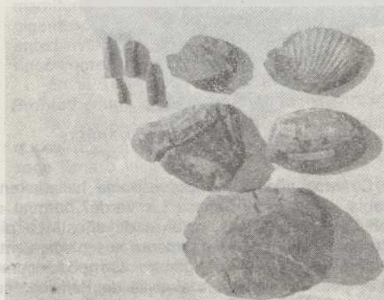
Fósiles de Peñalba
