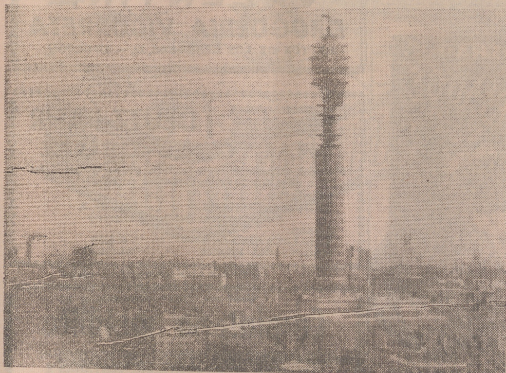
Sobresaliendo entre todos los edificios de Londres, vemos a la nueva torre de correos, que mide unos 174 metros de altura. En ella están instalados los servicios para la recepción y transmisión de enlaces con microondas para la Televisión y el servicio telefónico. Está recubierta totalmente de cristal y en su parte superior, cuando esté terminada, se montará un restaurante giratorio, que dará una vuelta completa cada media hora. — (Foto Fiel).
