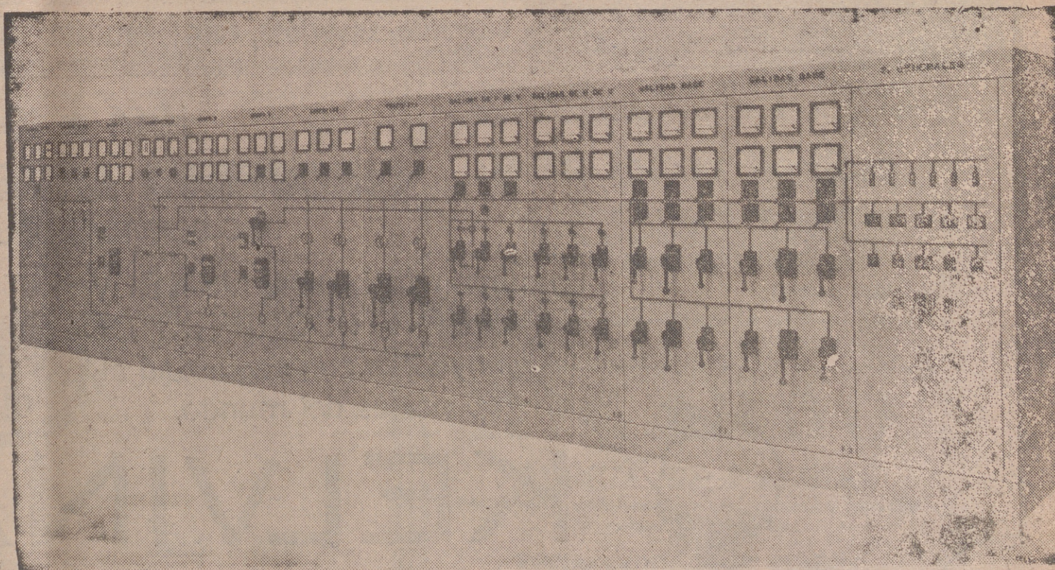
Cuadro de control y maniobra fabricado en la factoría de Ignacio Soria para la base aérea de Valencia (Zaragoza).
