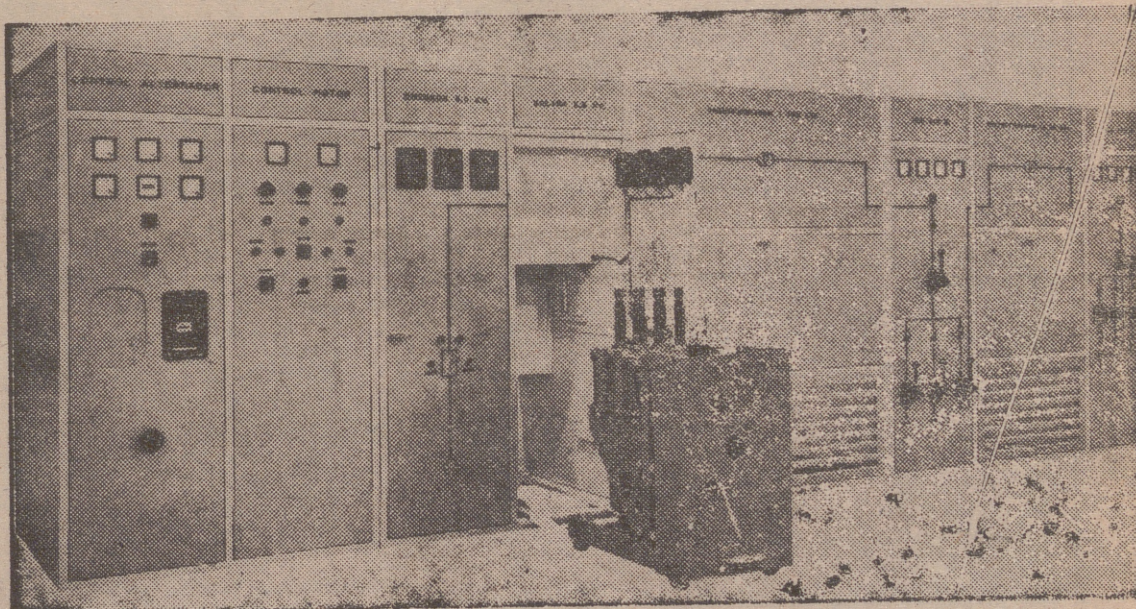
Isbloc para maniobra automática de central térmica, instalado por esta empresa, en Potasas de Navarra.
