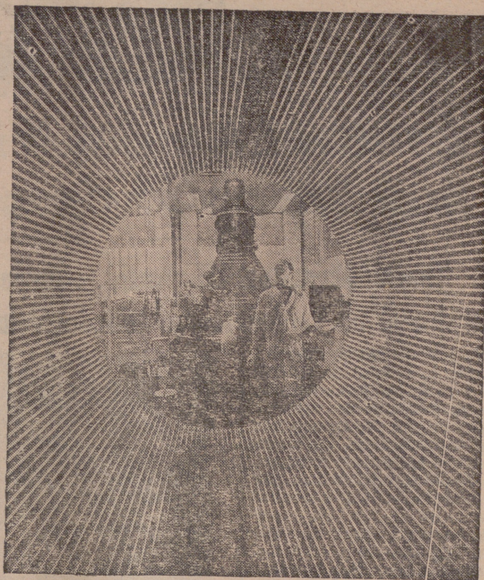
MOTOR LUNAR. —Los técnicos montan un motor F-1 en la fábrica que la North American tiene en Canoga, California. El motor está calculado para generar un empuje de 680.000 kilogramos. Un racimo de cinco motores F-1 integrará la primera fase del cohete Saturn V que se proyecta usar en el programa norteamericano Apolo de vuelo tripulado a la Luna. Esta fotografía ha sido tomada a través de una tobera de empuje del motor F-1.
