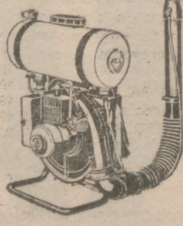
atomizador espolvoreador mínimo peso, largo alcance, polvo y líquido
