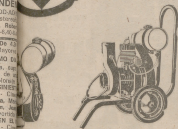
moto-bomba refrigeración por aire o agua grupos de 1, 2, 4 y 6 c.v.
