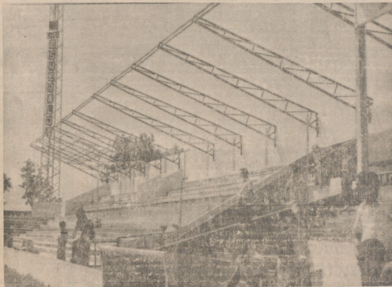
Este es el aspecto que va tomando la visera de la nueva tribuna. Las obras no pueden ir más rápidas. — (Foto Herce)
