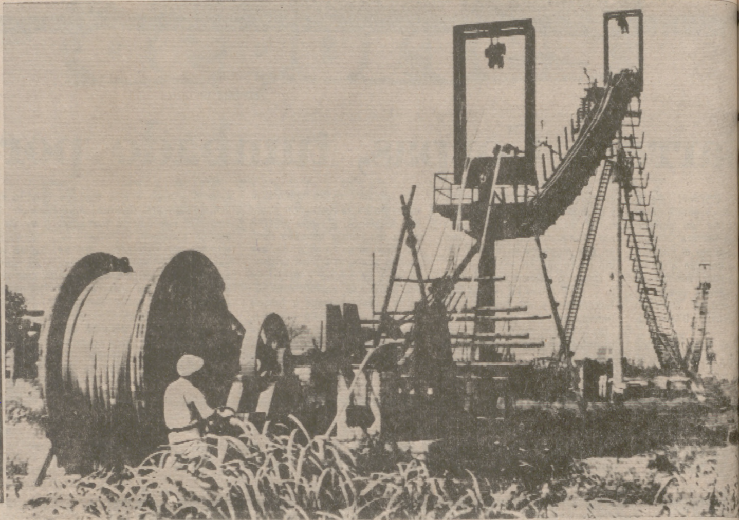
Un nuevo método de suspensión de puentes se prueba por vez primera en Japón. El método consiste en un grueso cable entre dos puertas en altura para sujetar el puente que va suspendido. Ciento cincuenta y ocho metros de puente cuestan por este método unos 140.000 dólares.
