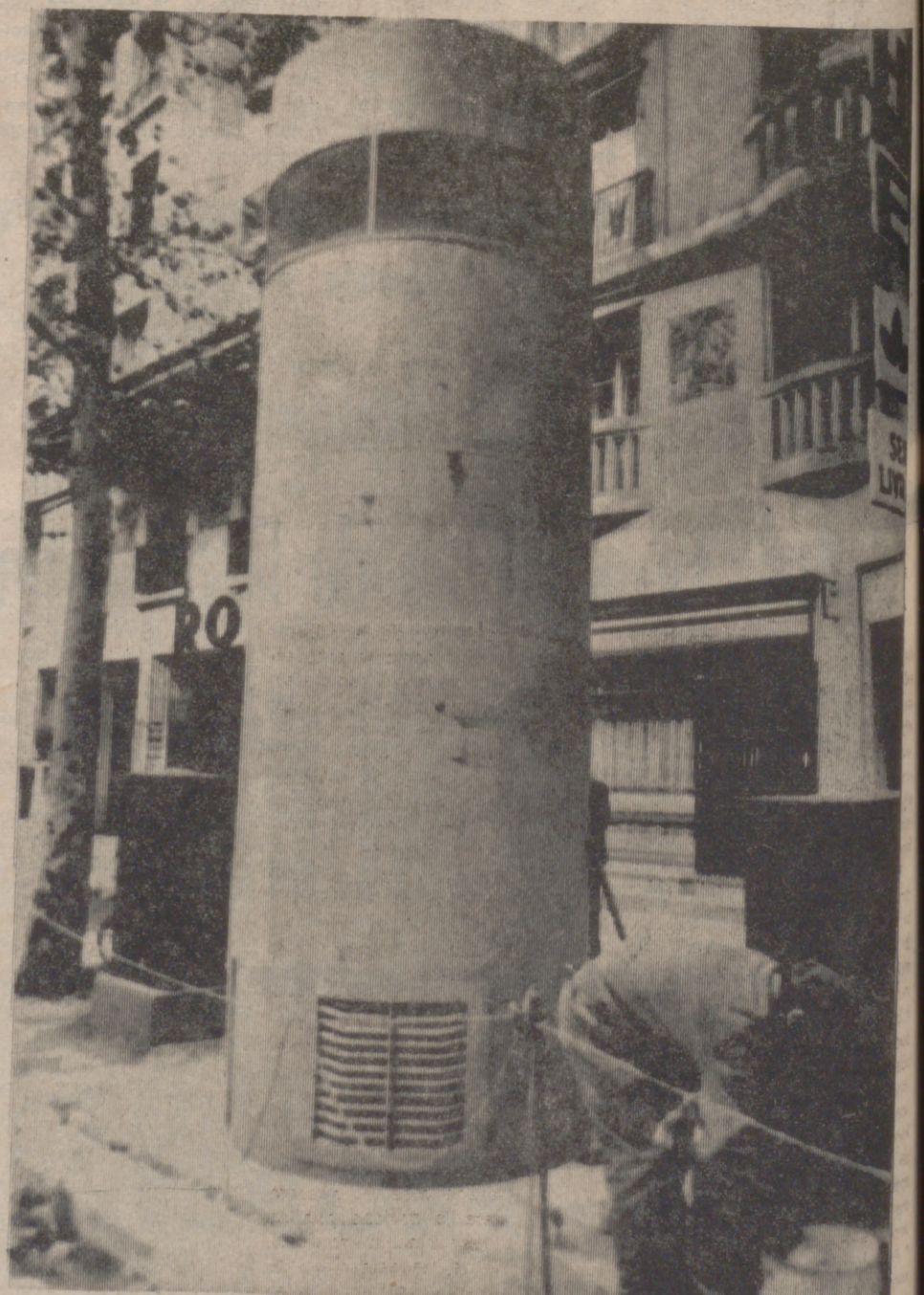
PARIS. — He aquí uno de los dos purificadores de aire que se instalan en la Avenida Rollin, de París. Tiene una altura de quince pies por cuatro y medio de diámetro. Consta de numerosos filtros en su parte superior. Tiene capacidad para depurar 330 millones de pies cúbicos al día. (Telefoto «Cifra Gráfica»)
