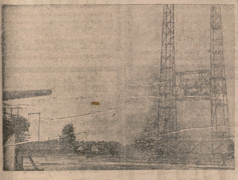
Cañones, tubos y pólvora son continuamente controlados para asegurar a los soldados alemanes las mejores armas. Con ayuda de este aparato, la marcha de la presión del gas en el tubo del cañón se fotografiada mediante un relojador y un oscilógrafo. (Foto Orbis)
