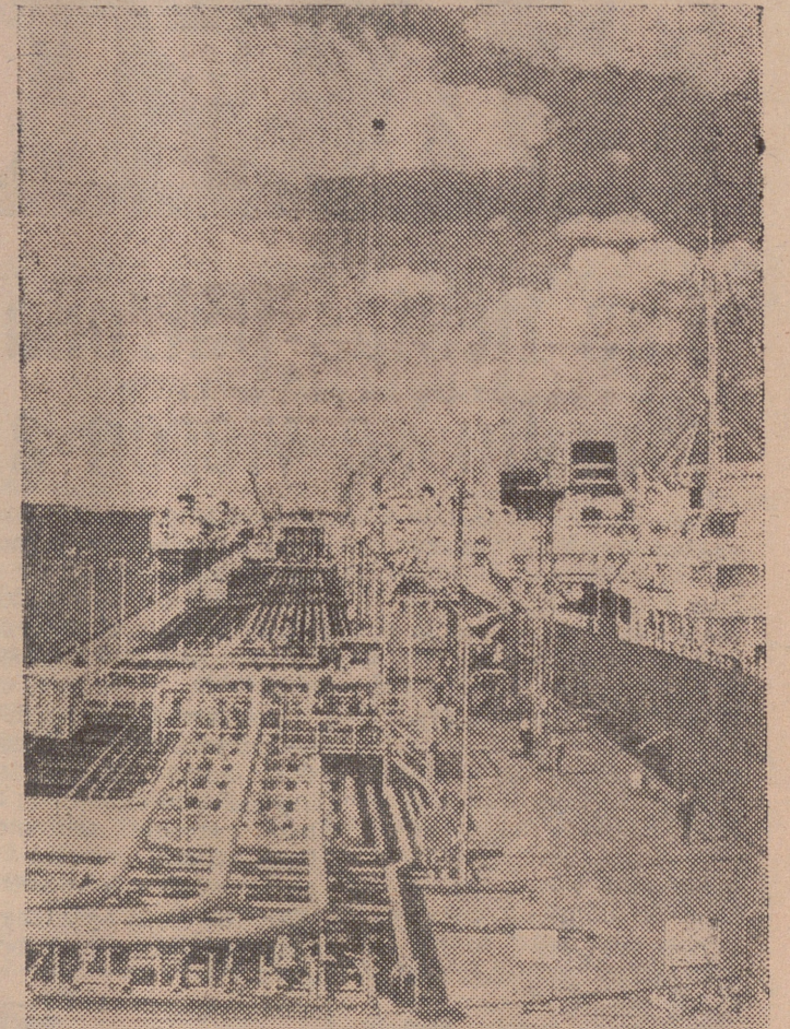
El final de los oleoductos que conducen al puerto de Mina Al Ahmadi (Kuwait), uno de los puertos petrolíferos mayores del mundo. La «Kuwait National Petroleum Company» ha propuesto al Gobierno de su país su asociación con el grupo petrolífero español «Hispanoil» para investigar y explotar la mitad del territorio nacional. (Foto Fiel)
