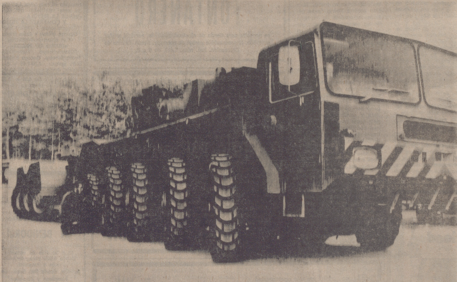
LAUF (Alemania). — El riesgo de pinchazo debe ser grande en un vehículo como ese, con diez ruedas en su parte delantera y seis en la plataforma posterior. Los ocho primeros responden a la dirección, como puede verse. Los otros ejes son fijos. El camión se utiliza como plataforma de una grúa gigante de un peso de 220 toneladas. — (Foto «Cifra Gráfica»).
