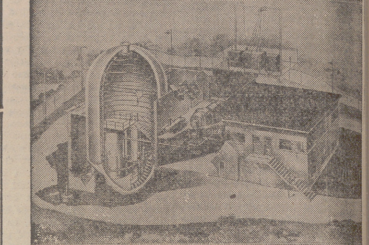
Dibujo a escala del reactor portátil del Ejército norteamericano, llamado así porque sus partes integrantes pueden transportarse por avión. Esta central portátil de energía nuclear será instalada en el Laboratorio de Investigaciones y Estudios de Fort Belvoir en Virginia.
