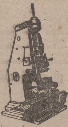
Mandrinadora para rectificar cilindros de 40 a 350 mm.
