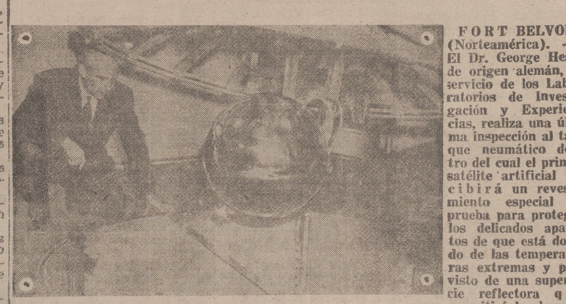
El satélite desde la Tierra. Los satélites del espacio forman parte del programa de participación de los Estados Unidos en el Año Geofísico Internacional. —(F. Cifra).
