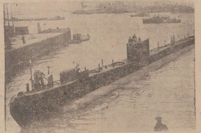
El "Explorer", submarino experimental británico de gran velocidad, entrando en el puerto de West Indian para una visita de seis días a Londres. El "Explorer", de 780 toneladas y 225 pies de largo, alimenta sus turbinas con vapor por medio de carbón "dióxido", y puede desarrollar toda su potencia cuando está sumergido.— (Foto Torremocha).
