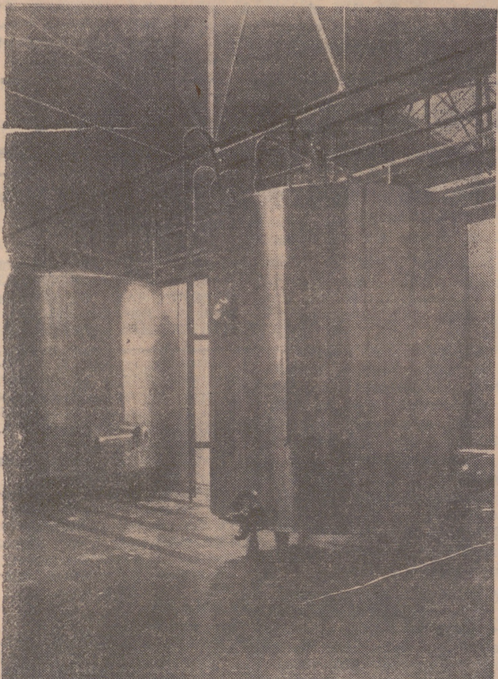
TANQUES DE RECEPCION DE LECHE DE 8.500 LITROS DE CAPACIDAD CADA UNO, CON DISPOSITIVO AUTOMATICO DE LAVADO
