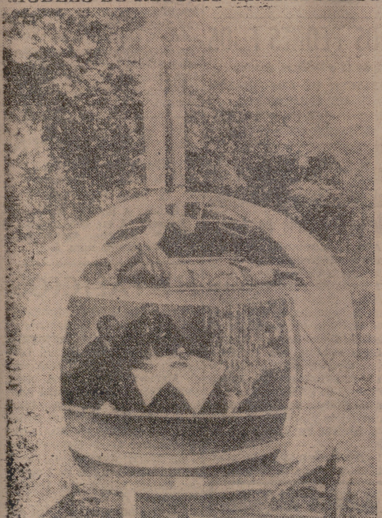
En una exposición celebrada en Hamburgo se exhibe este modelo de refugio antiatómico, proyectado por un ingeniero alemán. Es de acero y hormigón, puede contener hasta doce personas y sus paredes resisten presiones de hasta quince atmósferas. Su coste total será de unas 100.000 pesetas. (Foto Europa Press).
