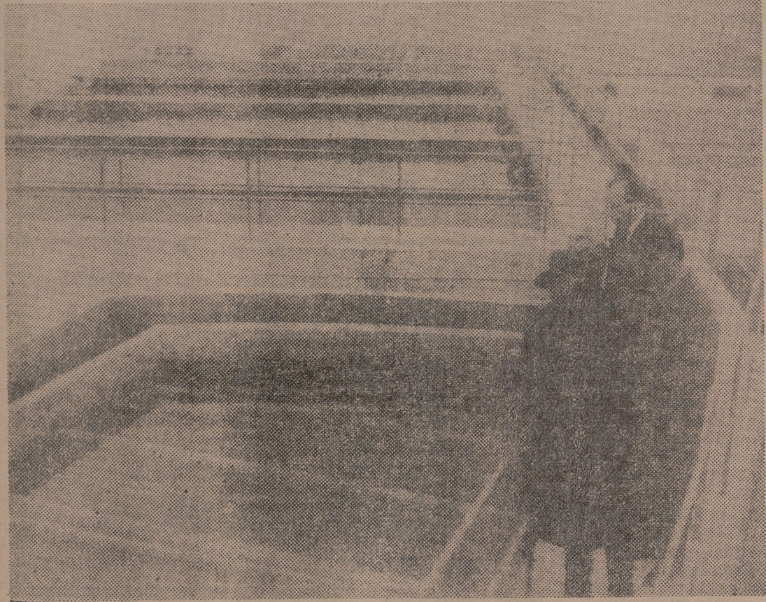
El señor Trevijano explica a los informadores locales el proceso de decantación en las nuevas instalaciones de la traída de aguas.
