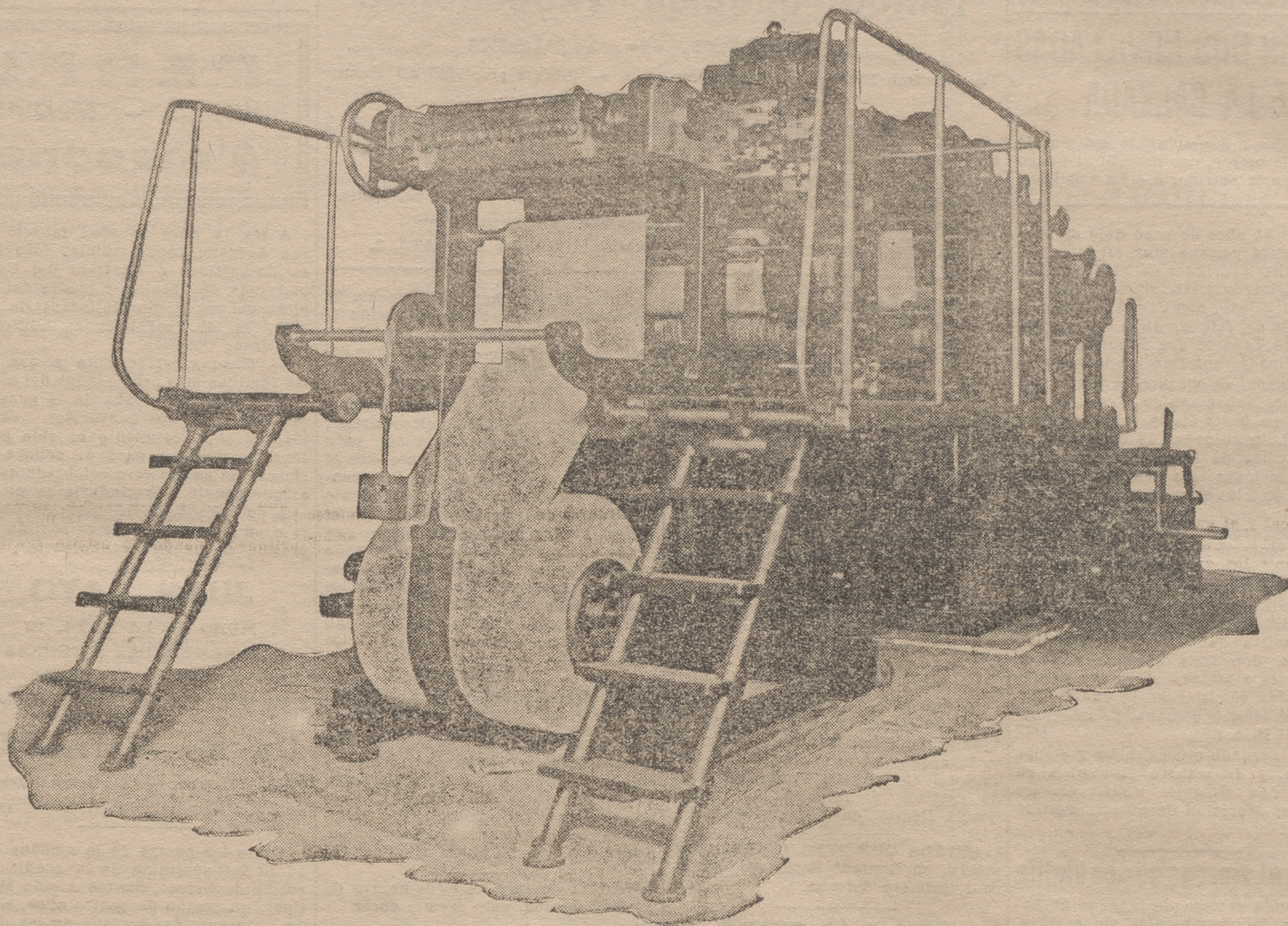
La rotativa de LA RIOJA, de la Casa alemana Alibert, dotada de una ampliación construida por la Razón social LEIZAOLA, S. L., de San Sebastián
