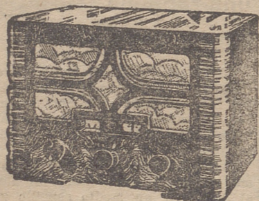
821 A.—SUPER-OCTODO, corriente alterna, ondas cortas y largas. Precio: 485 ptas.
