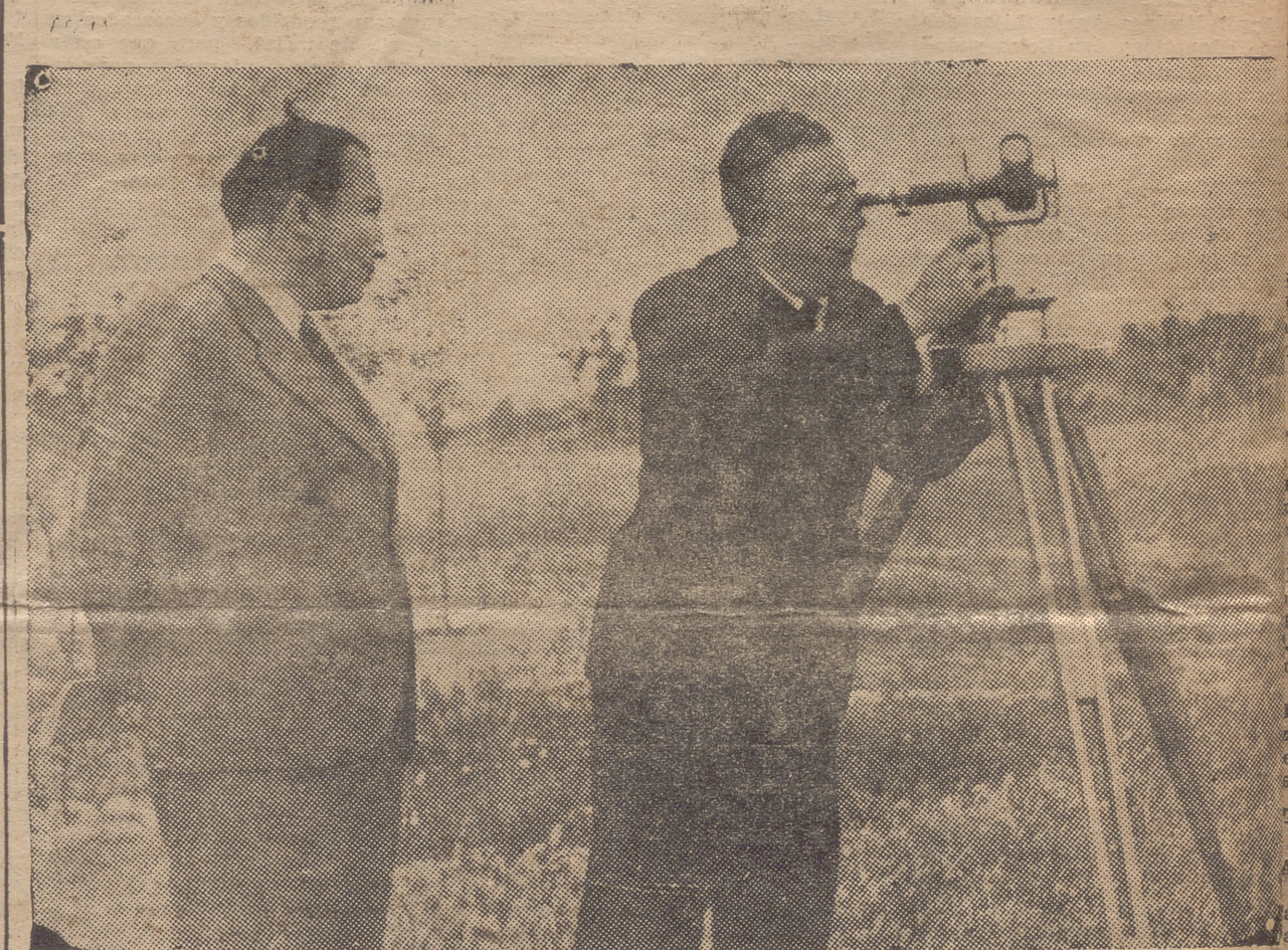
EL DIRECTOR DEL OBSERVATORIO SIGUIENDO CON EL TEODOLITO LA MARCHA ASCENSIONAL DEL GLOBO
