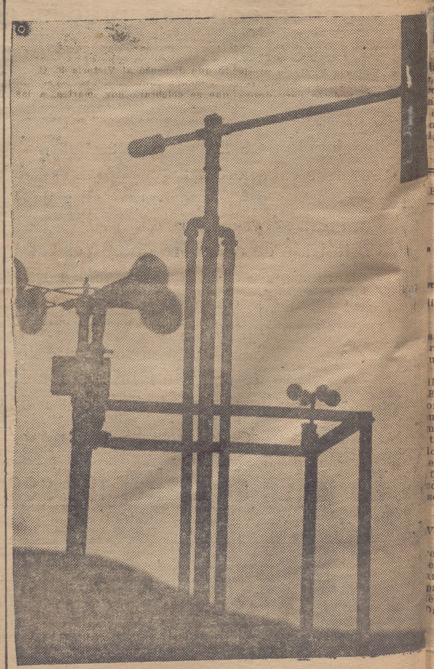
LOS ANEMOMETROS Y LA GRAN VELETA, TOMADOS A SU ALTURA
