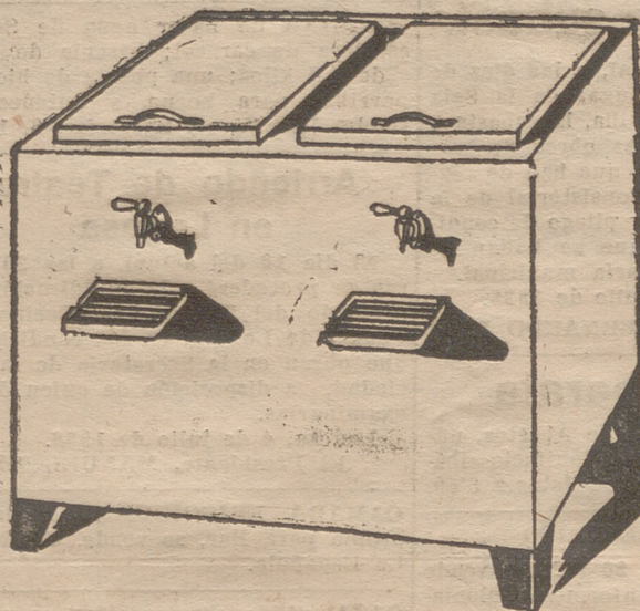
Modelo para pequeños Bares, Hoteles, etc. Cabida: 100 botellas. Producción, 2 kgs. de hielo cada vez. 2 serpentines y 2 grifos para cerveza y agua. PTAS. 3.500.
