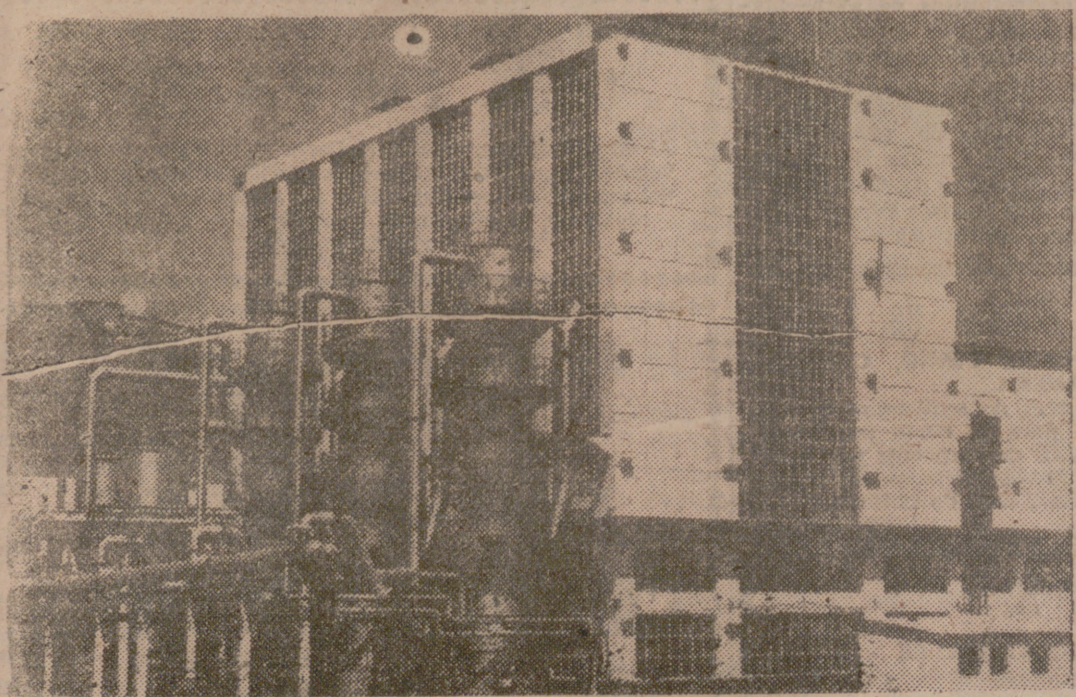
PUENTES DE GARCÍA RODRÍGUEZ (Coruña).— Edificio de gasificación y torres de lavado del gas de dicha fábrica, dependiente de la Empresa Nacional Calvo Botello.— (Foto Cifra).
