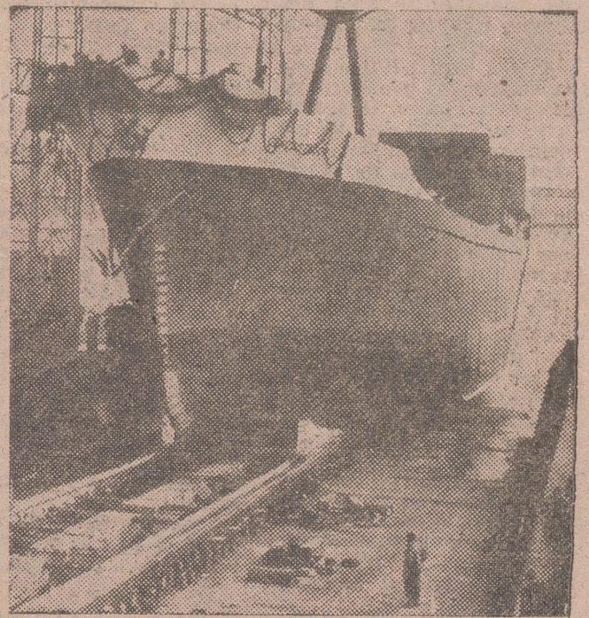
SEVILLA. — Momento de la botadura del buque «Conquistador», construcción número 39, realizada en los astilleros de Sevilla de la Empresa Nacional «Elcano» y con destino a la Naviera Alvargonzález. Este buque es gemelo de otro botado en junio pasado. — (Foto Cifra).
