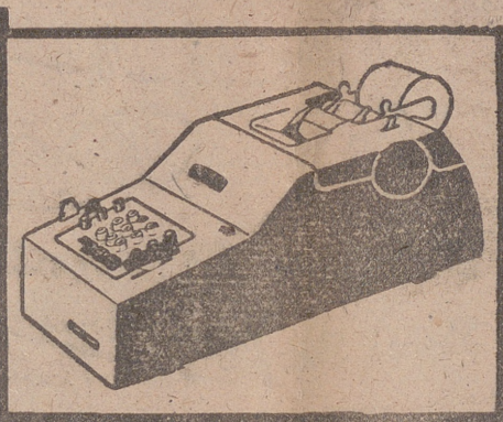
Electrosoma
