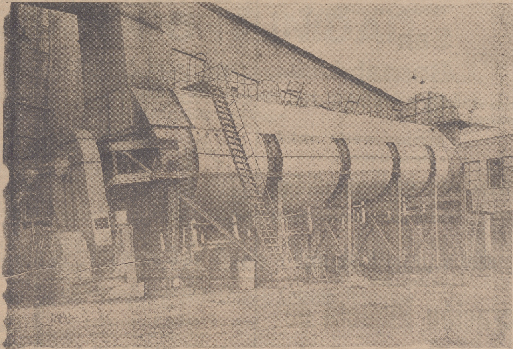
Difusión de la Casa danesa "De Danske Sukkerfabrikker" instalada por su licenciataria en España, S. A. JULIANA CONSTRUCTORA GIJONESA, en Azucarera del Duero
