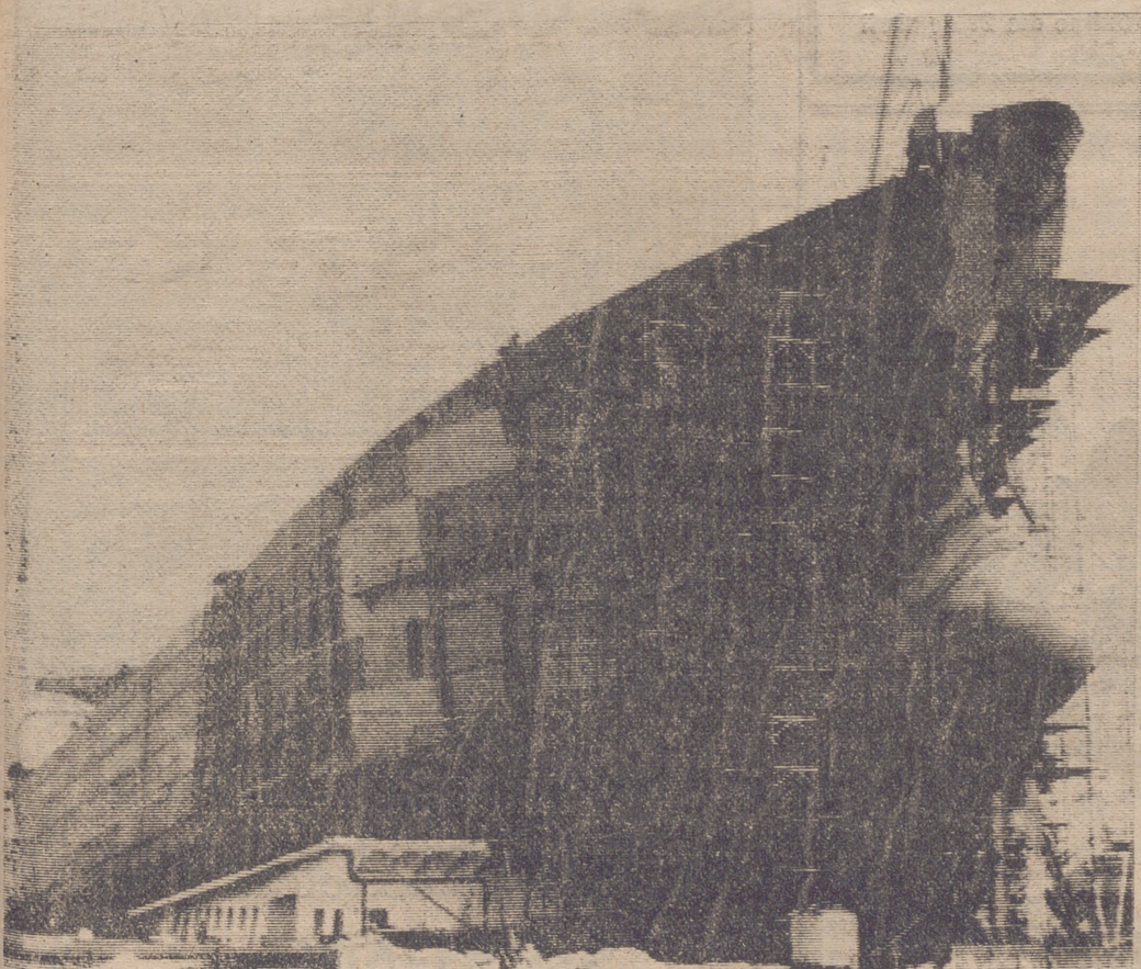
El próximo mes de mayo será botado en los astilleros gaditanos el mayor petrolero construido hasta la fecha en España. Tiene 243'95 metros de eslora, 35'50 de manga y 16'70 de puntal, y un peso muerto de 66.600 toneladas. La proa ha sido construida con una característica especial que se denomina "de bulbo". En la foto le vemos en los astilleros, donde se le están dando ya los últimos toques. Este es el primero de una serie de tres que serán construidos. --- (Foto "Fiel").
