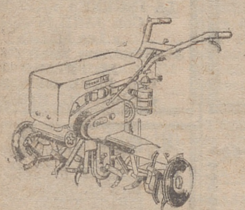
MOTOAZADAS DE 35-6 y 7 C.V.
