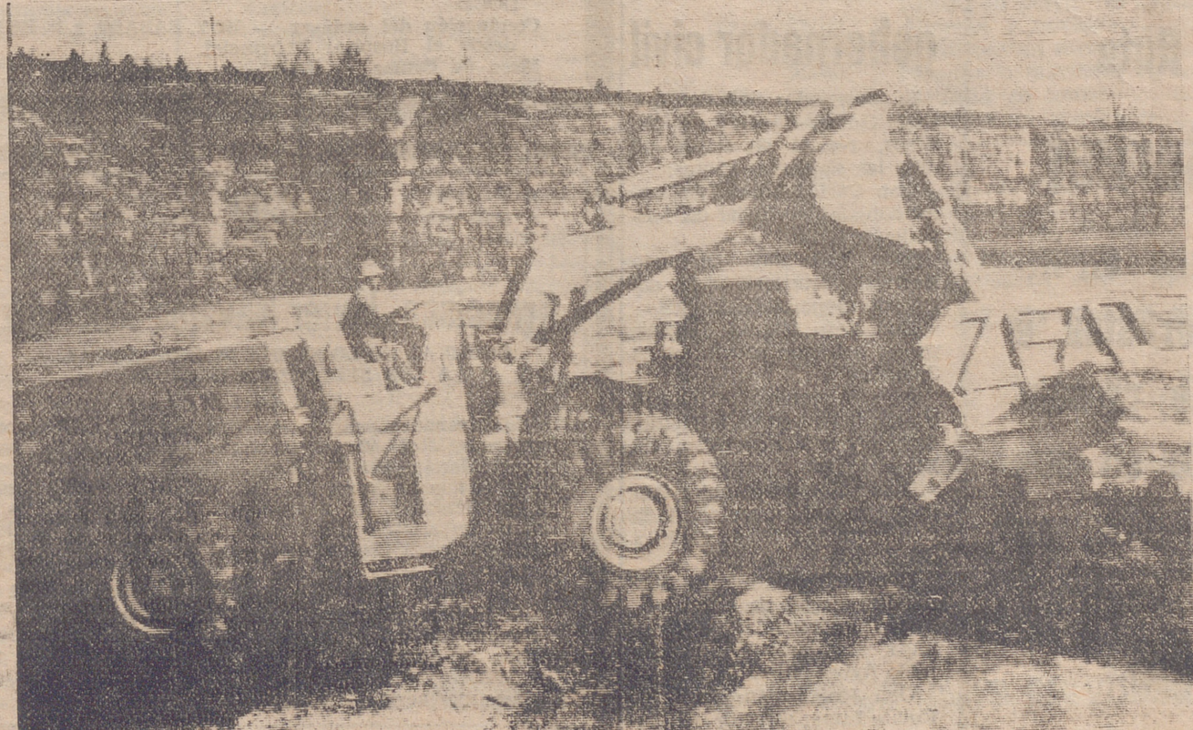
La máquina modelo "4900", de doble articulación, es la mayor Pala Cargadora del mundo
