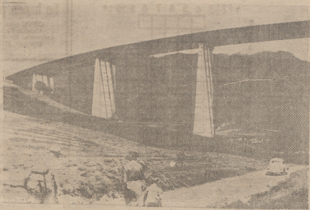
Sobre suelo austriaco se está construyendo la autopista del Brenner. Muchos valles y cañadas son salvados por puentes elevados como el de esta fotografía, cerca de Steinach, en los Alpes. Se espera que para dentro de tres años esté terminada esta importante vía de comunicación. — (Foto "Fiel").
