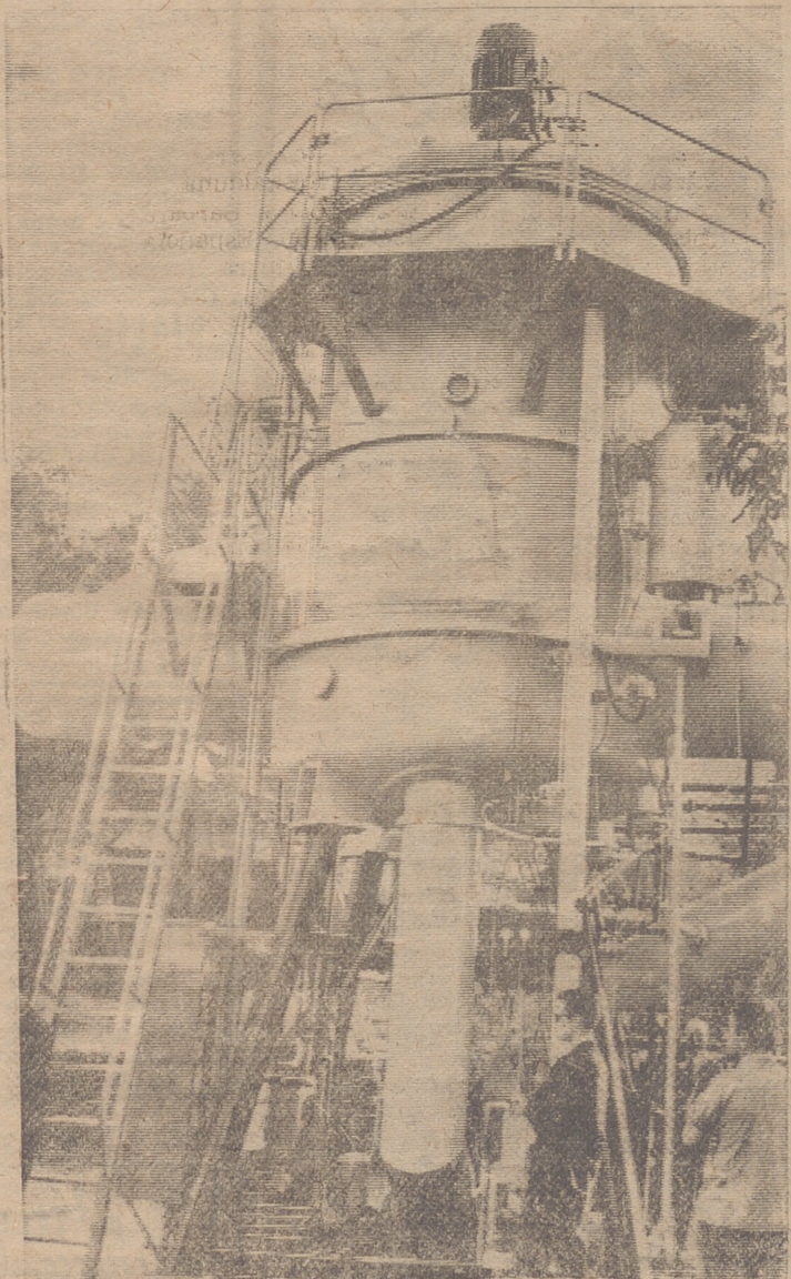
Ha sido bendecida e inaugurada en Cadaqués, en plena Costa Brava, una moderna planta desalinizadora de agua del mar, segunda de España y primera de la Península, ya que solamente existe otra en las Islas Canarias, siendo a la vez, al parecer, la primera del continente europeo. Así, pues, en Cadaqués ya no tendrán problema de agua. — (Foto "Fiel").
