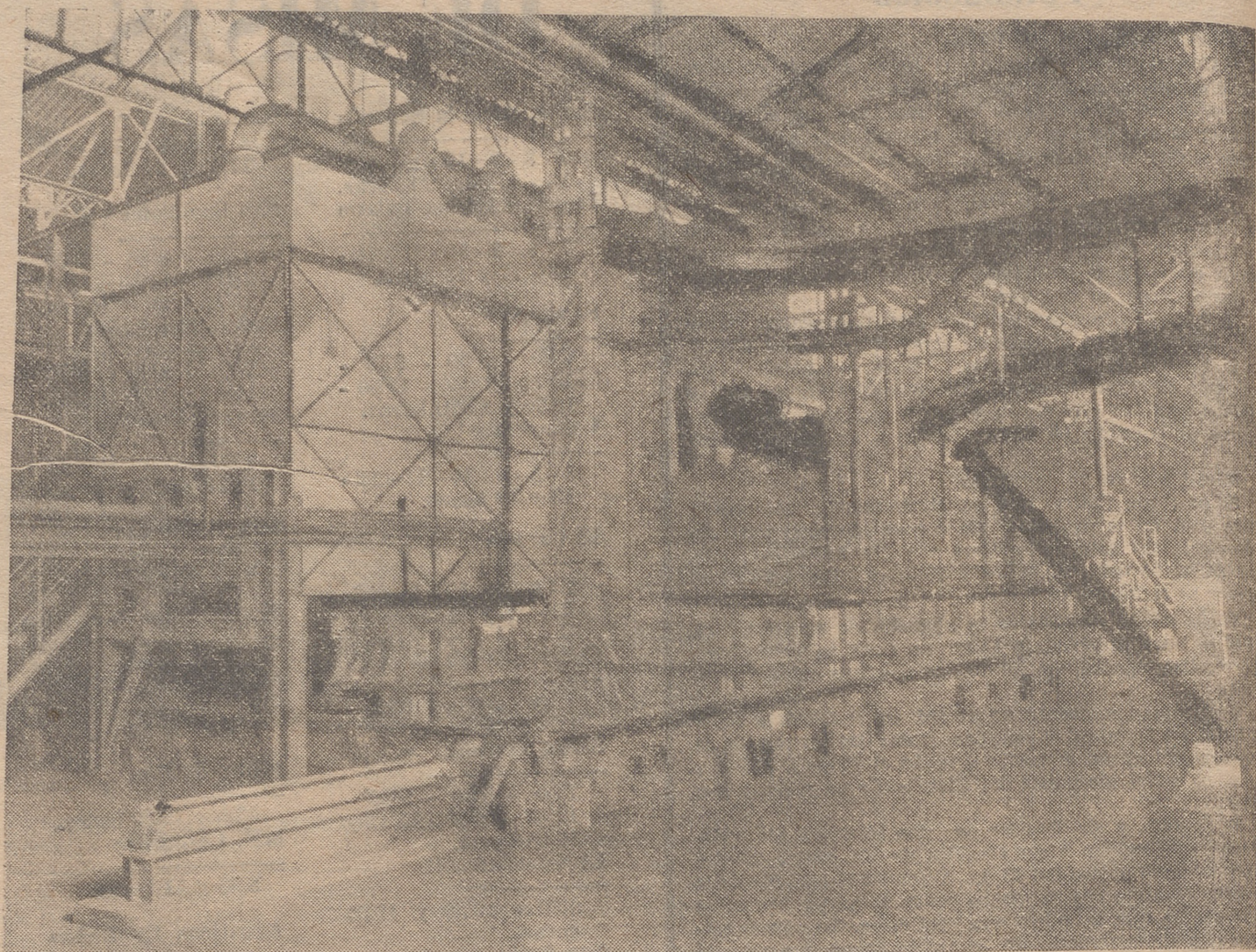
Vista parcial de la más moderna factoría automática de bañeras de hierro fundido del mundo, con capacidad para producir una bañera cada cuarenta y ocho segundos.
