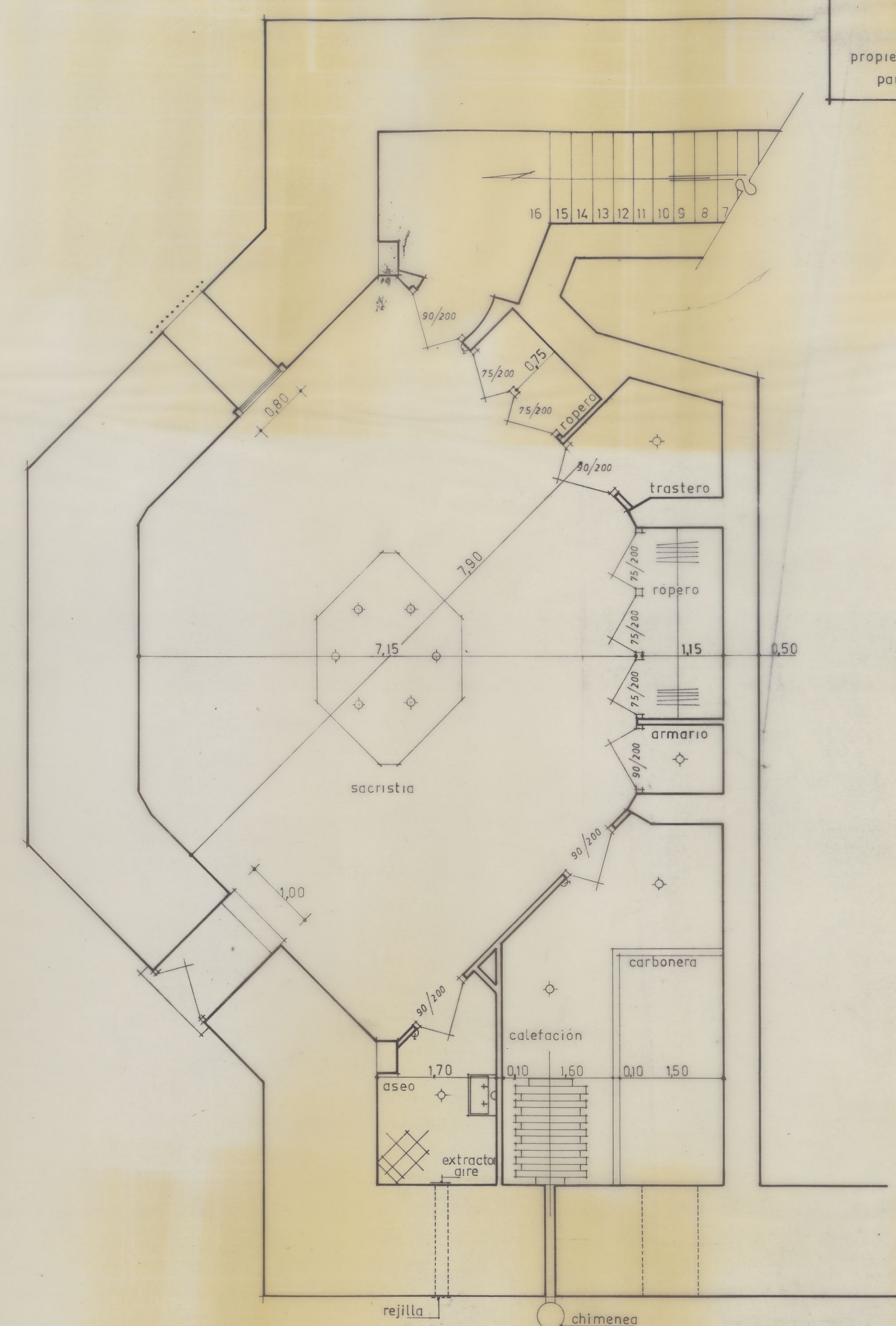
Planta sacristía
