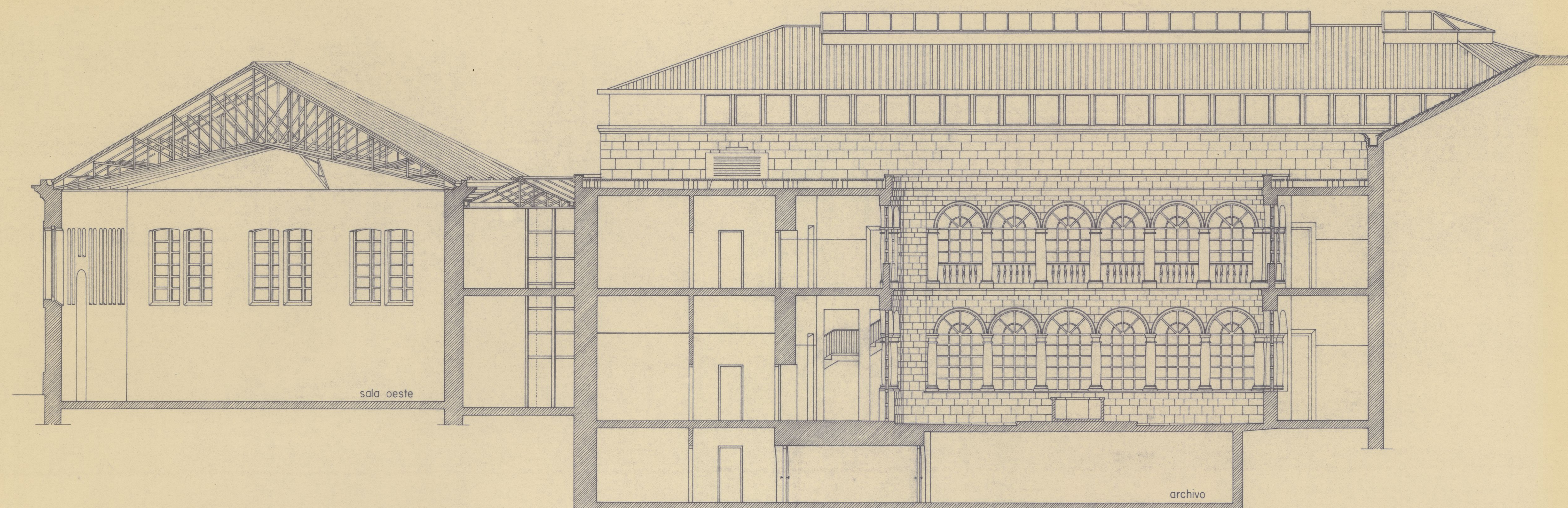
Sección A.A
