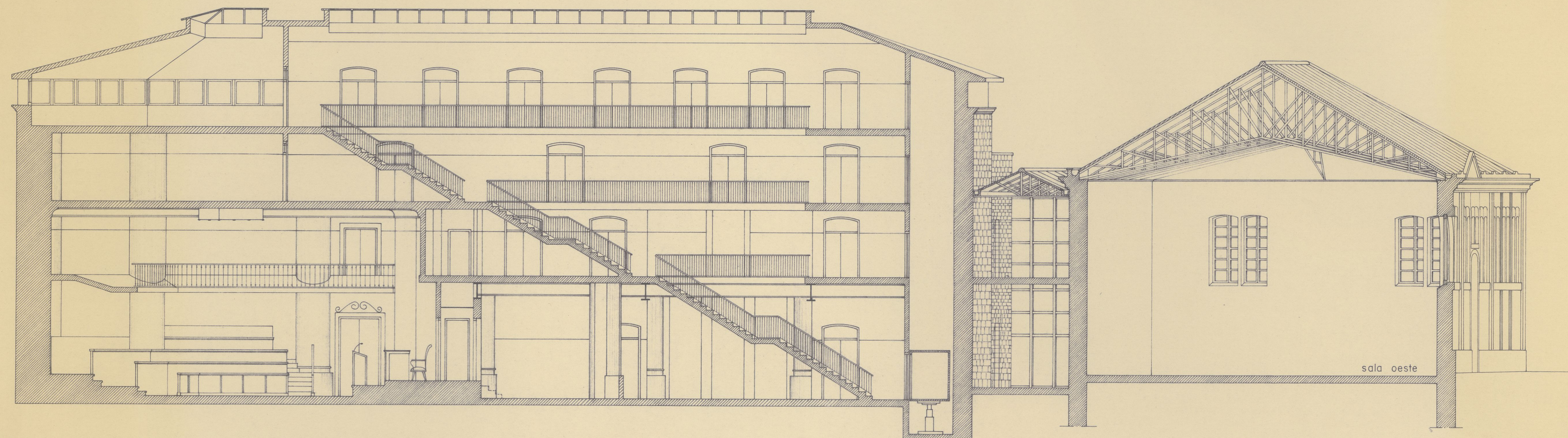
Seccion CC
