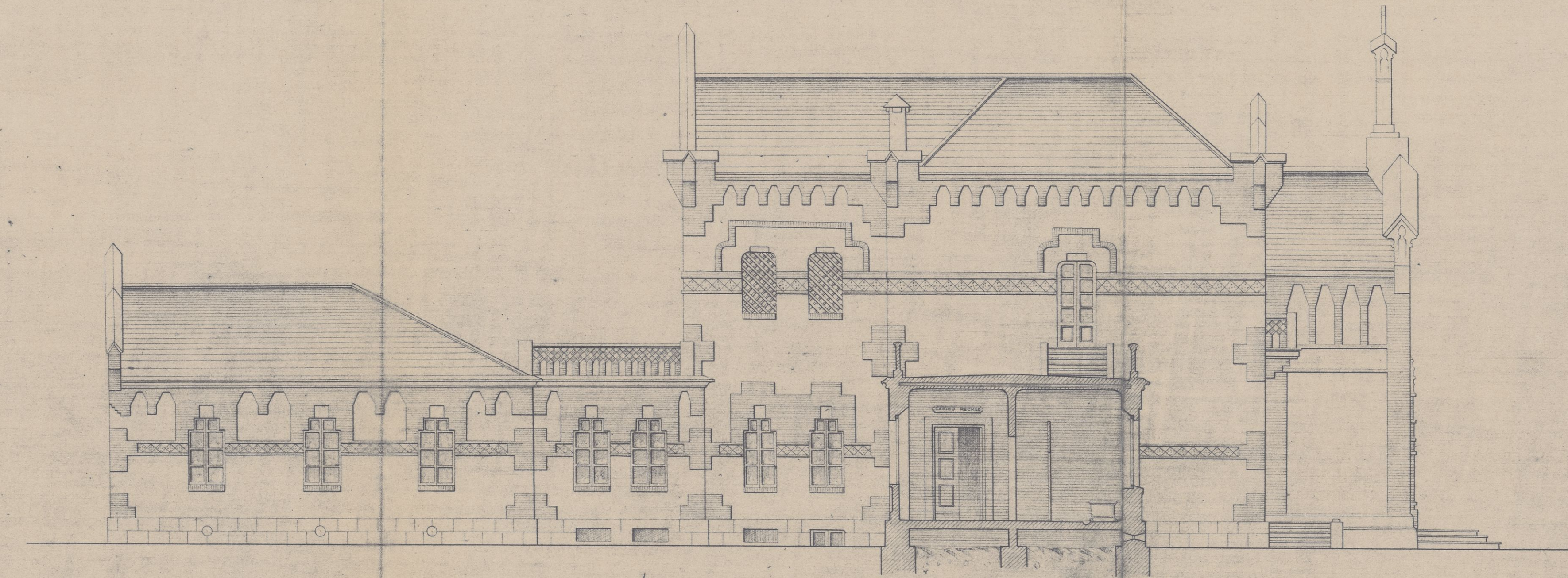
Sección por CD Escala 1:100
