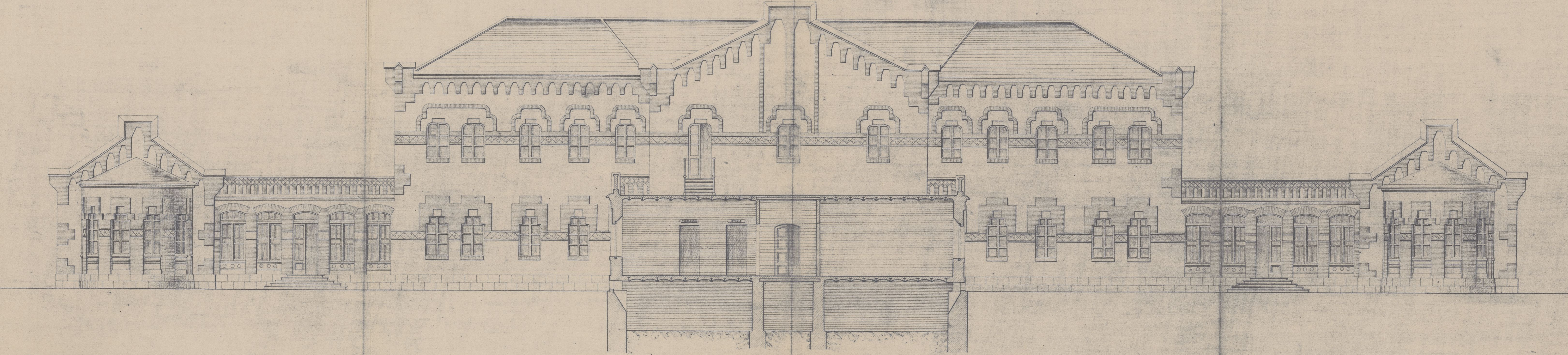
Sección por EF Escala 1:100
