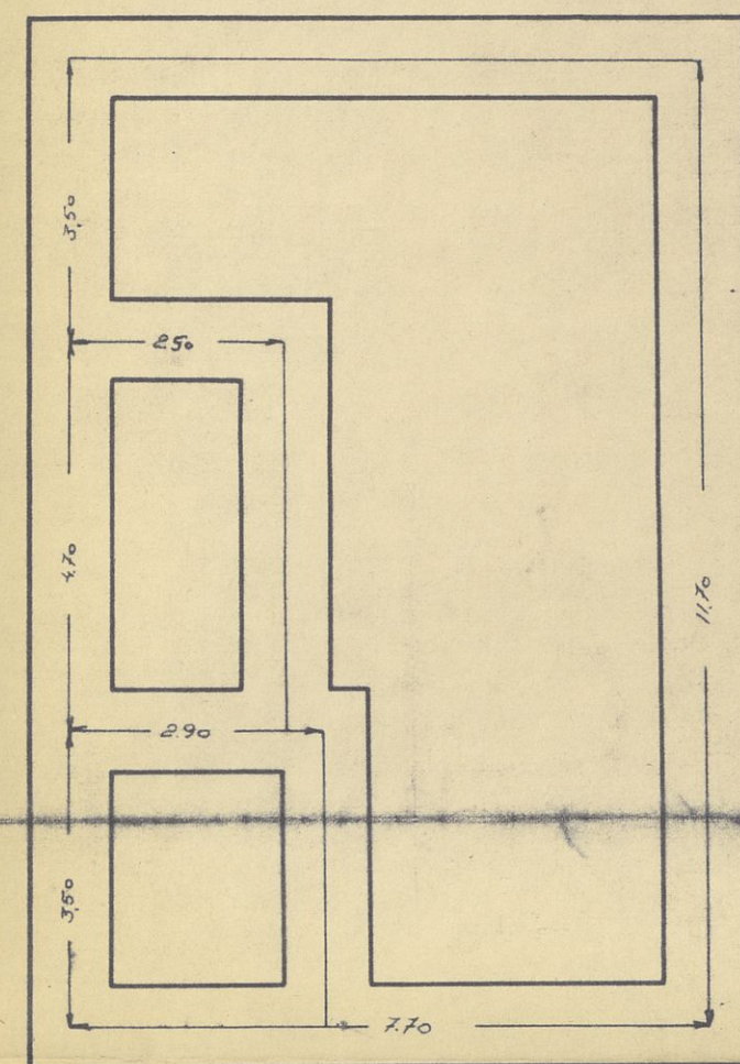
PLANTA de CIMIENTO
