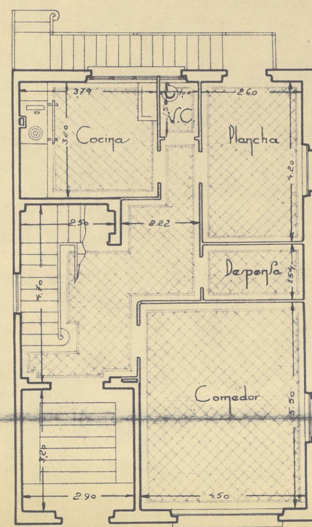
PLANTA de ENTREUSO
