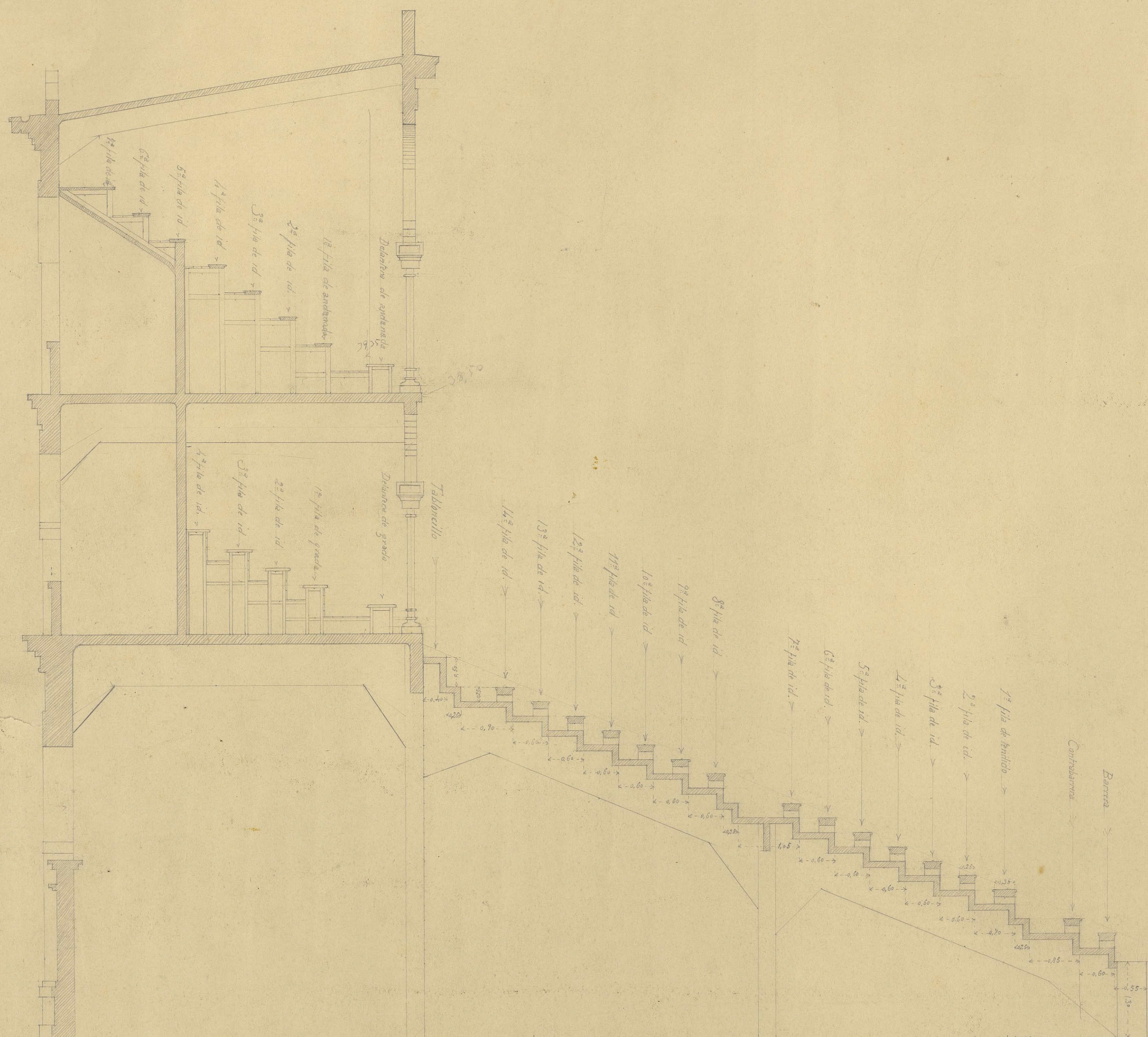
SECCION DE GRADERIA DE TENDIDO, GRADA Y ANDANADA. ESCALA 1:50
