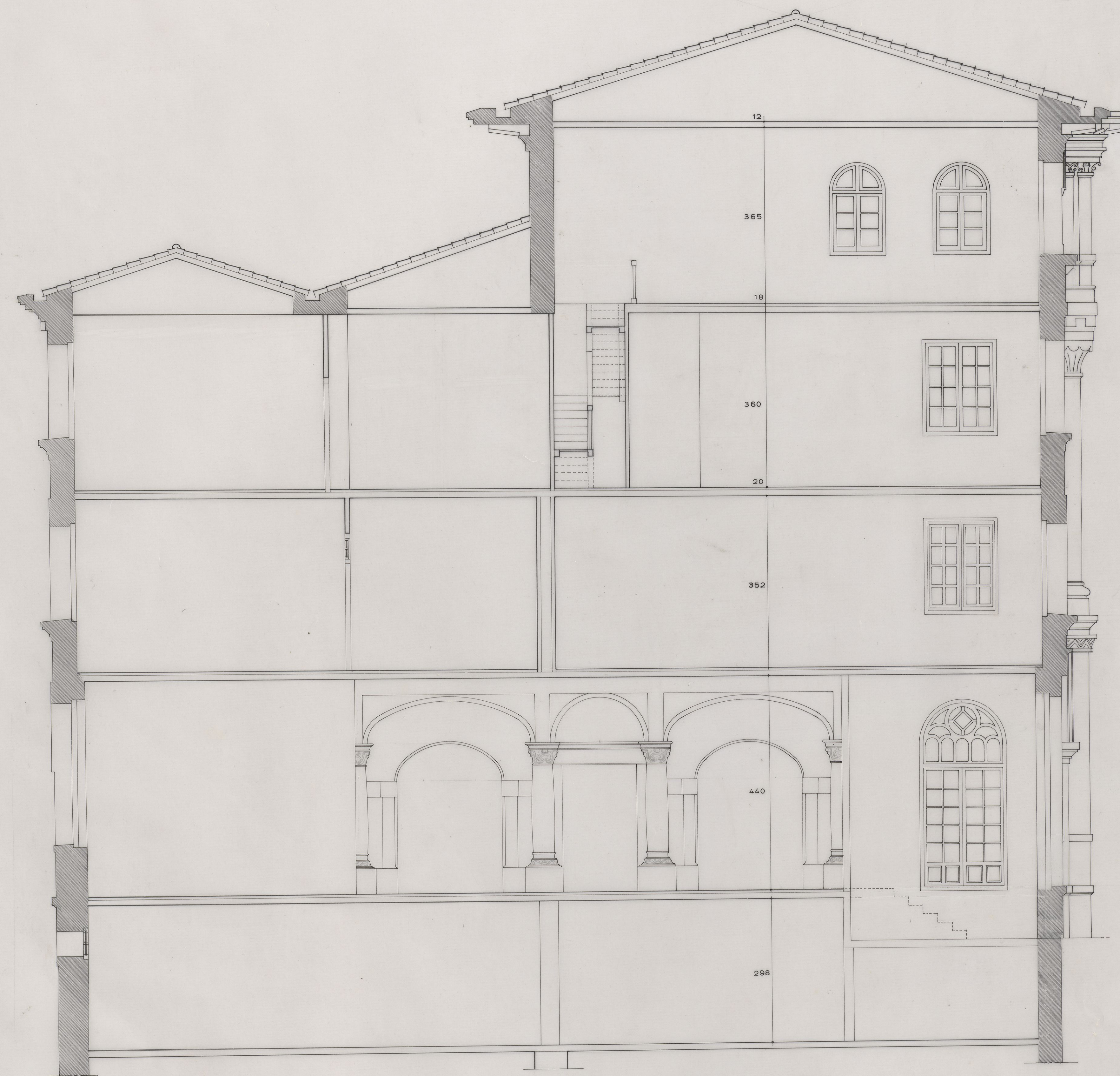
SECCION: 2. (estado actual).
