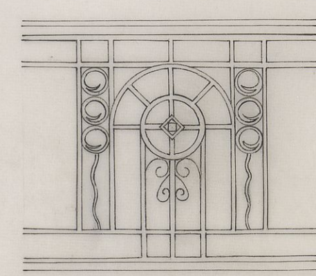
DETALLE BALAUSTRÉ ESCALA 1:20
