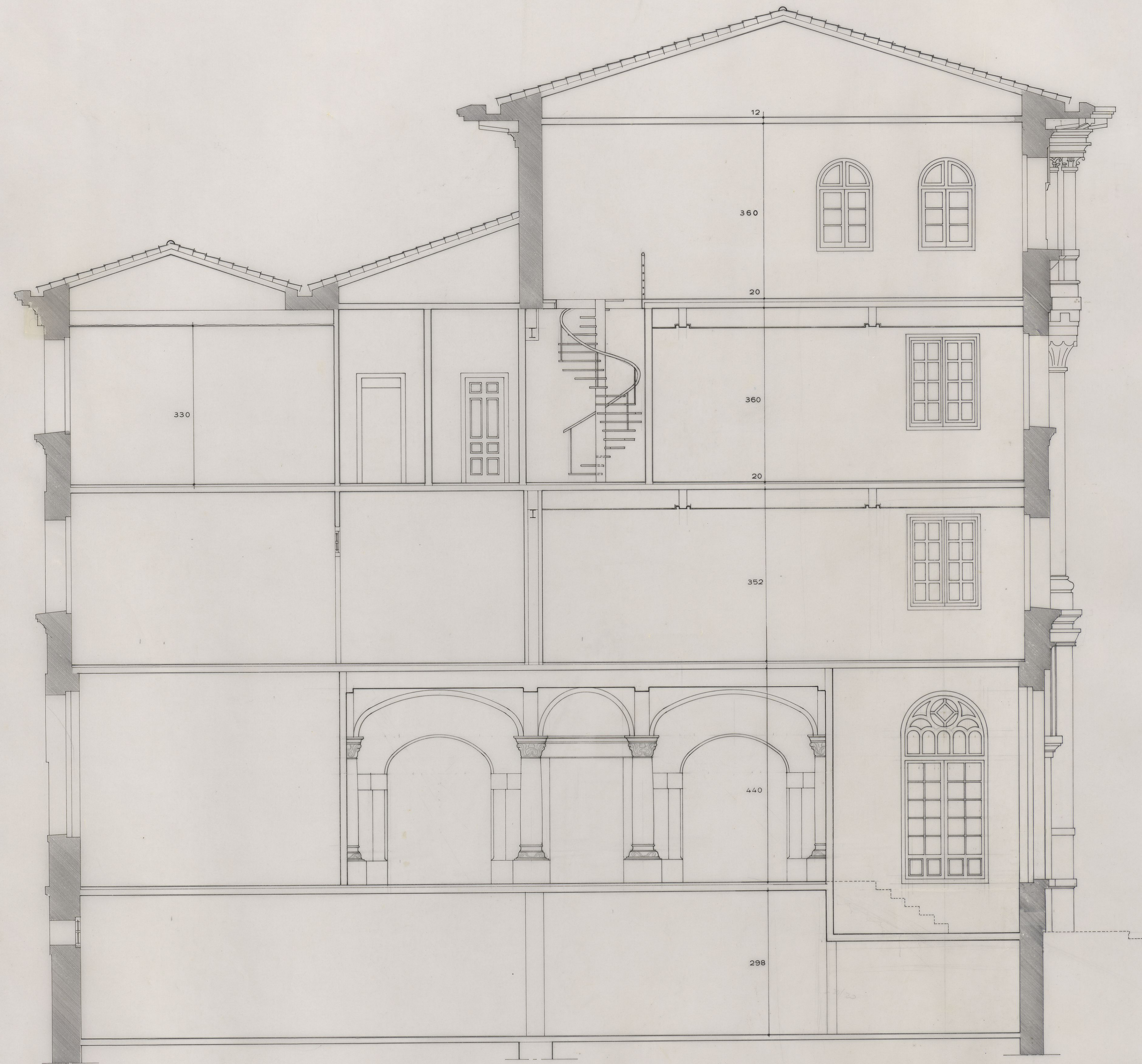
SECCION:- 2. (estado reformado).
