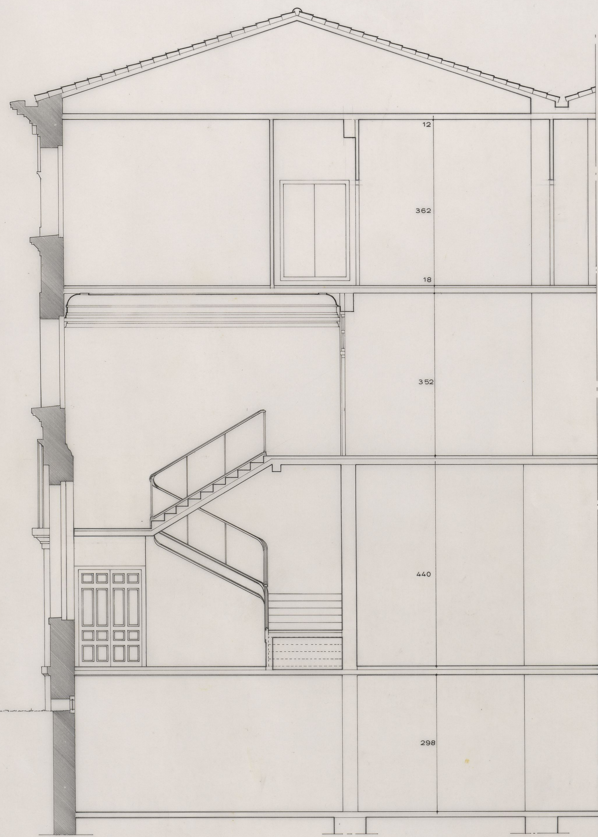
SECCION.- 1.-1'
