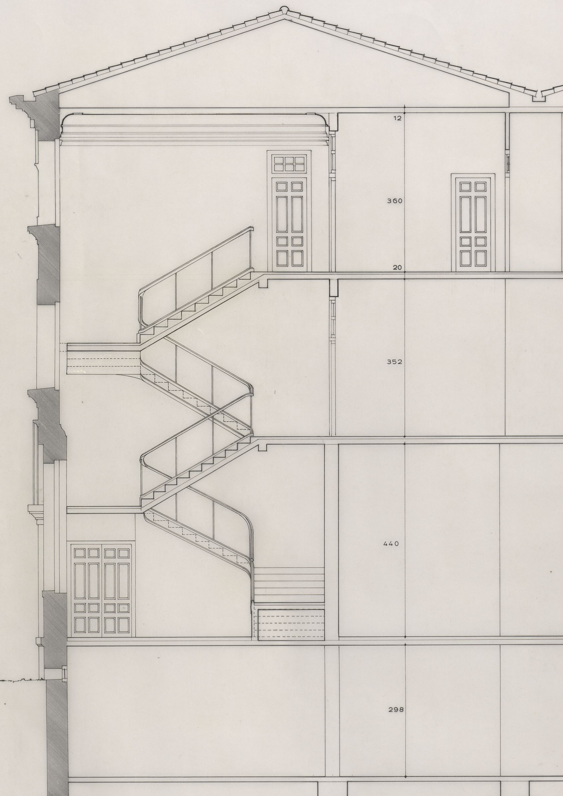
SECCION:- 2-2'
