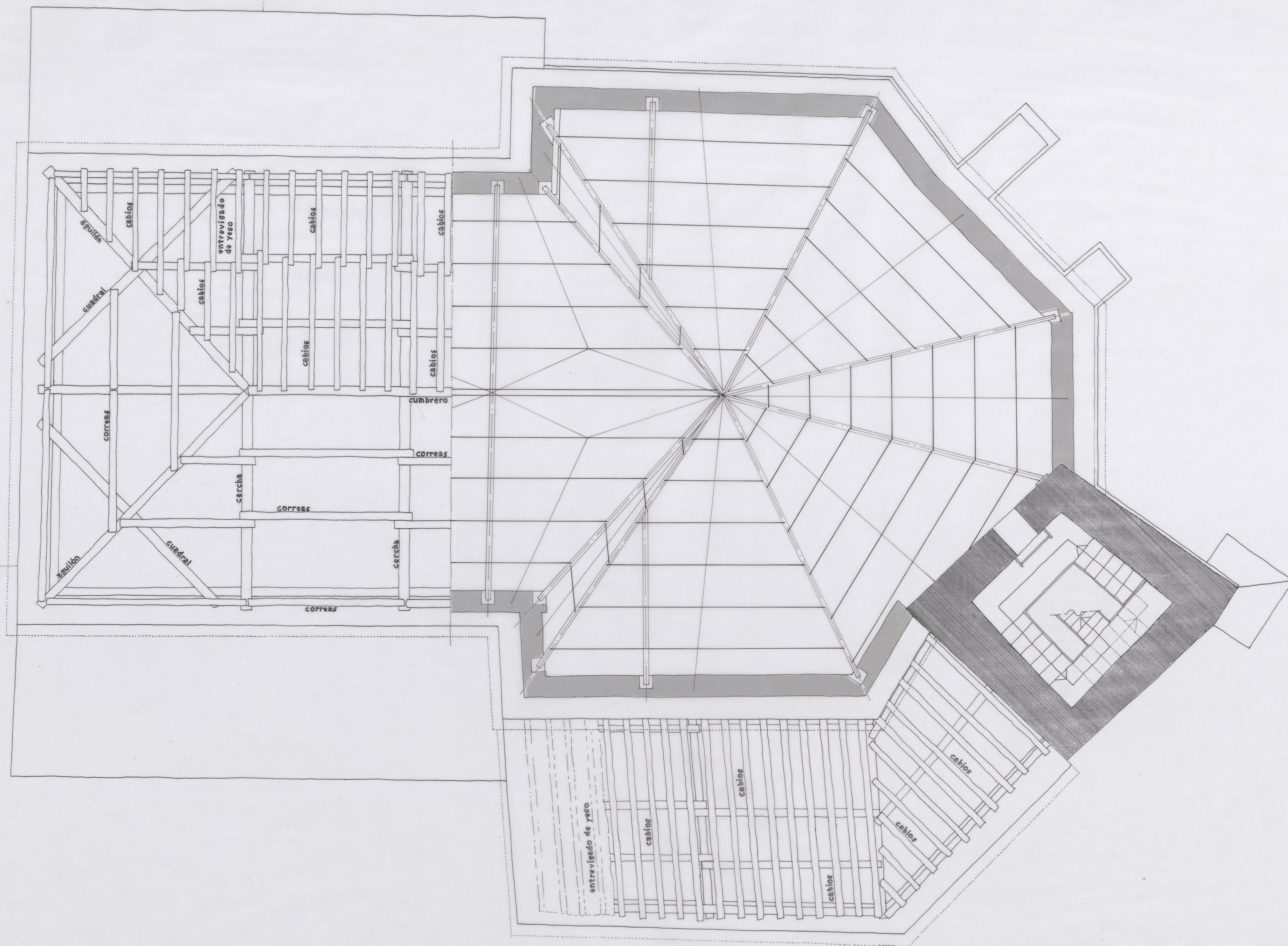
PLANTA DE ESTRUCTURA DE CUBIERTA (en zona de actuación.)
