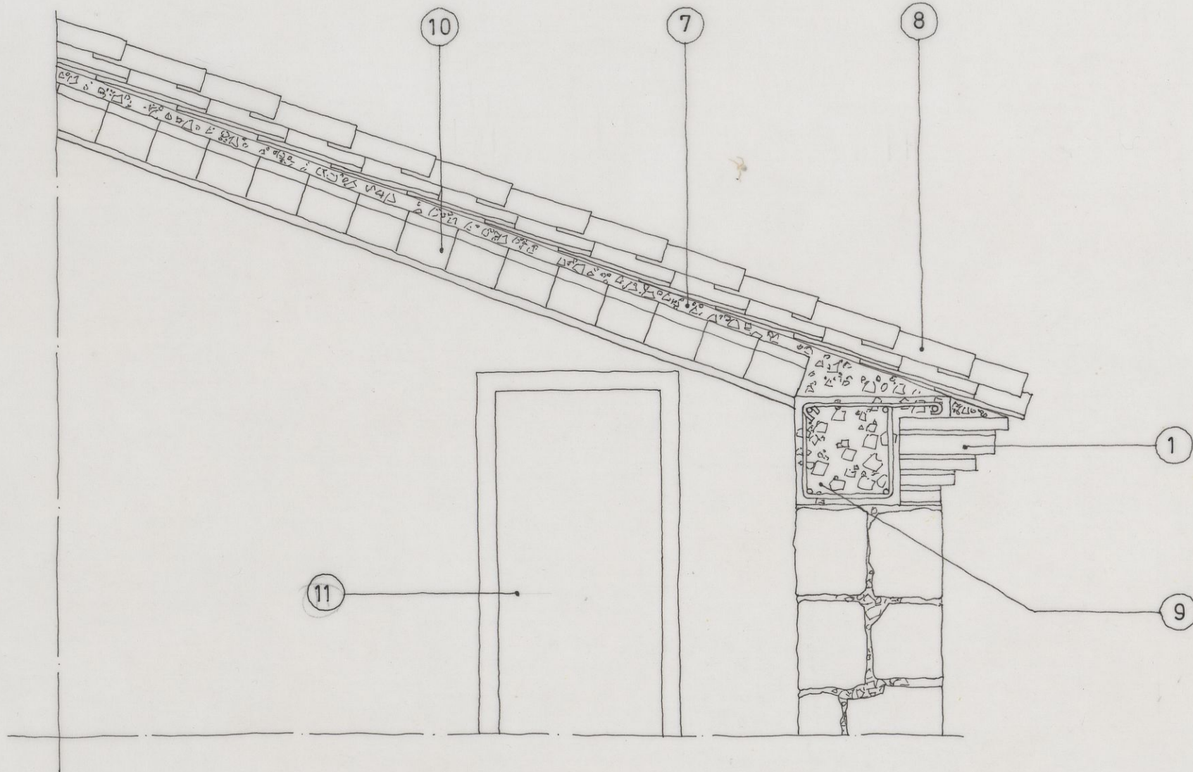
DETALLE CONSTRUCTIVO EN ZONA DE ACCESO A TORRE (E = 1/20)
