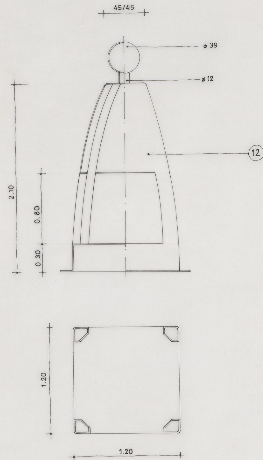
DETALLE DE REMATE CUBIERTA TORRE (E = 1/25)
