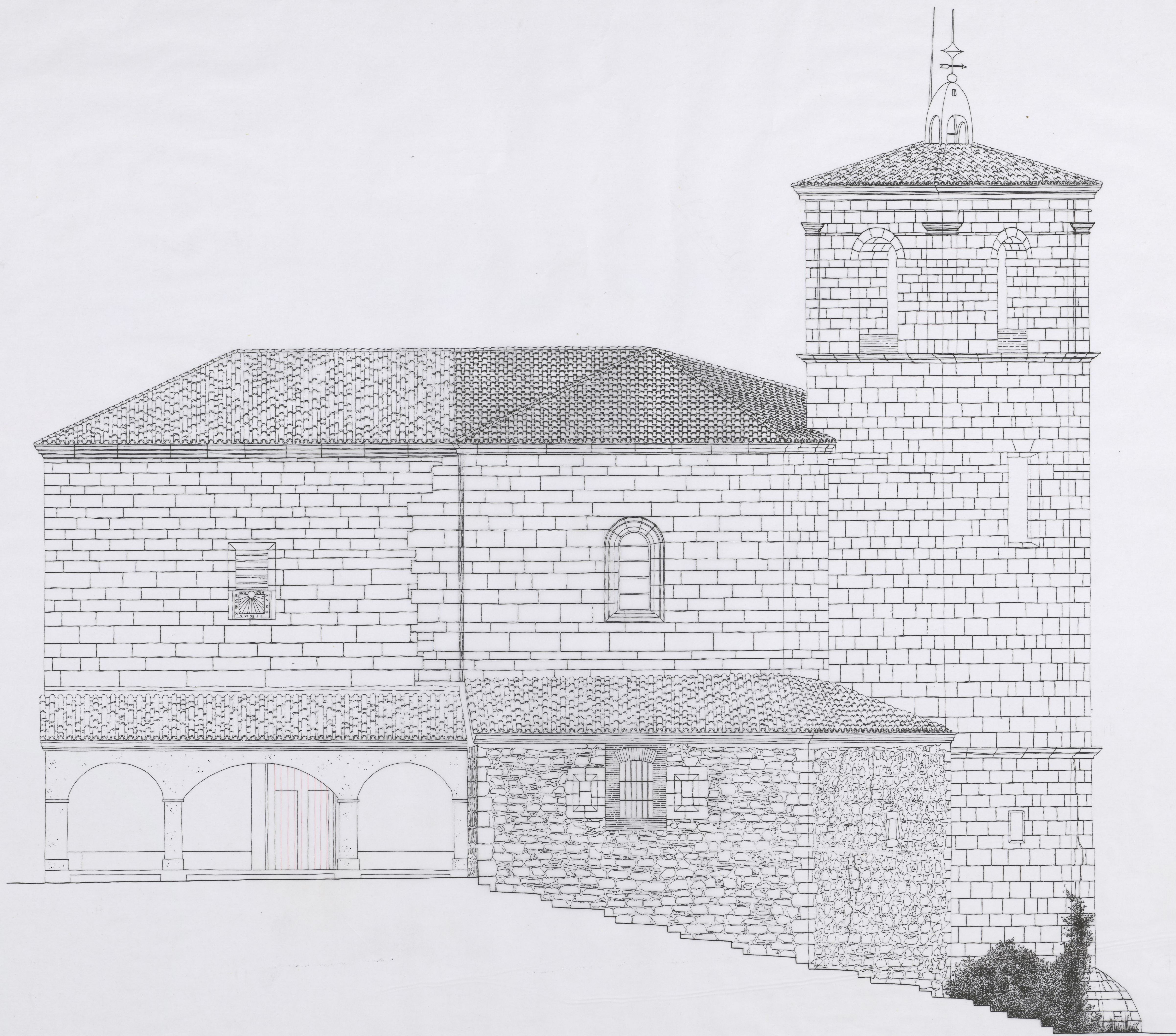
ALZADO SUR
