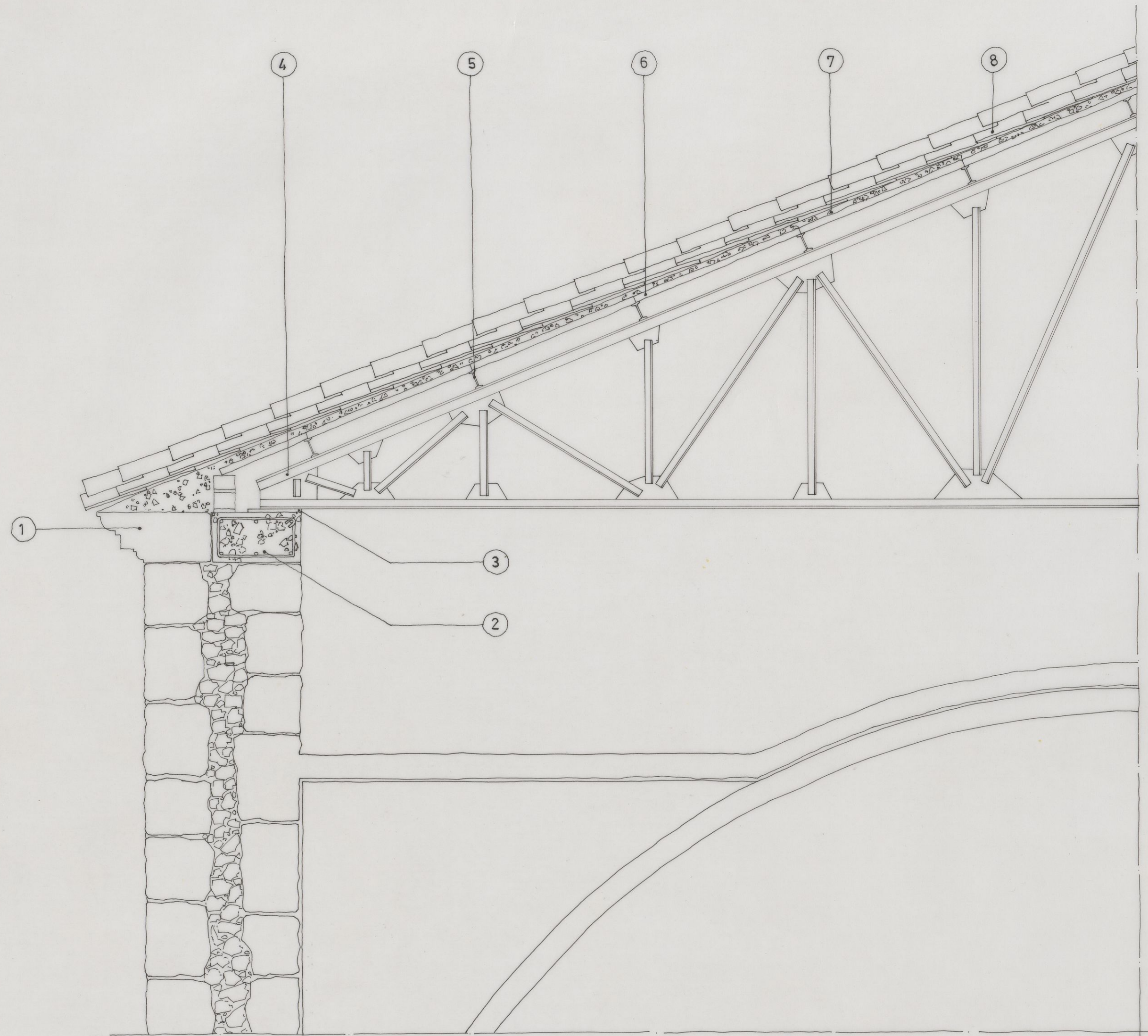
DETALLE CONSTRUCTIVO DE CUBIERTA EN ZONA DE NAVE CENTRAL (E = 1/20)
