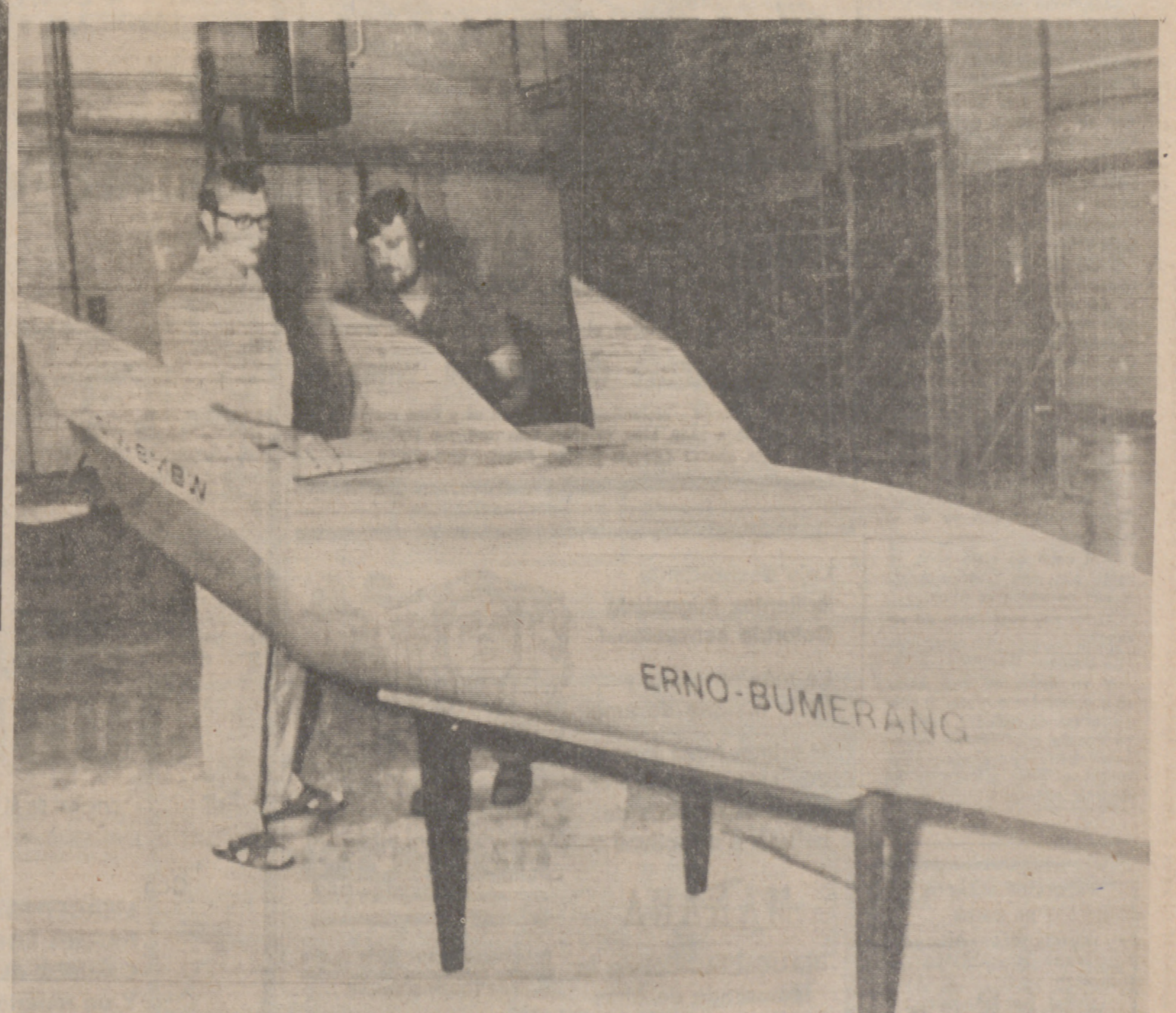
BREMEN (Alemania). — Esta es la maqueta de un futuro aparato de vuelo para la reentrada de los astronautas en la atmósfera terrestre desde una estación espacial. El «LB 23 Boomerang» ha sido diseñado por Erno Space Technique Company para la NASA y será construido para utilizarlo también como planeador sobre la Tierra. La primera prueba de vuelo con esta maqueta, de 3,10 metros de longitud por 1,90 entre alas y 400 kilos de peso, se realizará mañana sobre el Mar del Norte. Este modelo será llevado por un avión de transporte «Tranzall» de la Fuerza Aérea Alemana. — (Telefoto «Cifra Gráfica»).
