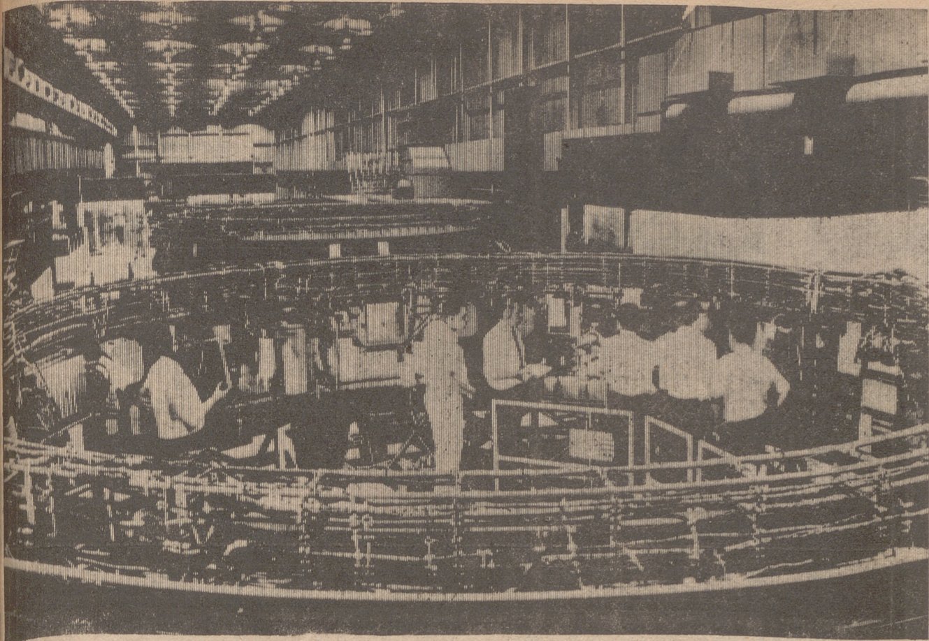
La Unidad de Instrumentos, construida y montada por IBM en su Centro de Sistemas Espaciales de Huntsville, Alabama, es una de las secciones más importantes del cohete impulsor Saturno V, que pondrá en órbita al "Apolo 11". En esta unidad se alojan 57 dispositivos (equipos electrónicos, eléctricos y mecánicos para la guía, navegación y control, y sistemas de medición y telemetría de los datos de funcionamiento y ambiente) además de las fuentes energéticas y el equipo de control ambiental para refrigeración. La unidad dispone además de un ordenador digital, con sus circuitos por triplicado, diseñado y construido por IBM en Owego, Nueva York. En esta foto vemos un momento del montaje de tan complicada e importante fase del cohete. --- (Foto Fiel).
