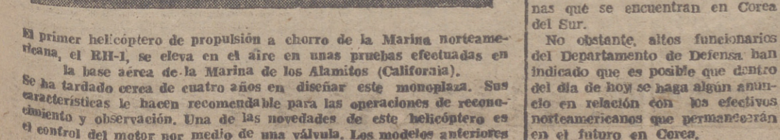
El primer helicóptero de propulsión a chorro de la Marina norteamericana, el RH-1, se eleva en el aire en unas pruebas efectuadas en la base aérea de la Marina de los Alamitos (California). Se ha tardado cerca de cuatro años en diseñar este monoplaza. Sus características le hacen recomendable para las operaciones de reconocimiento y observación. Una de las novedades de este helicóptero es el control del motor por medio de una válvula. Los modelos anteriores solo disponen de «encendido» y «apagado».
