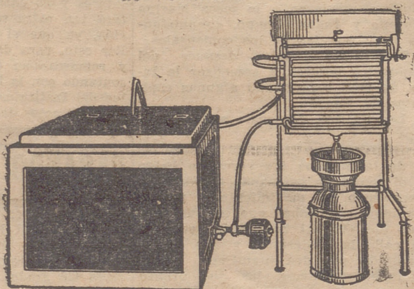
Instalación enfriadora y conservadora de leche
