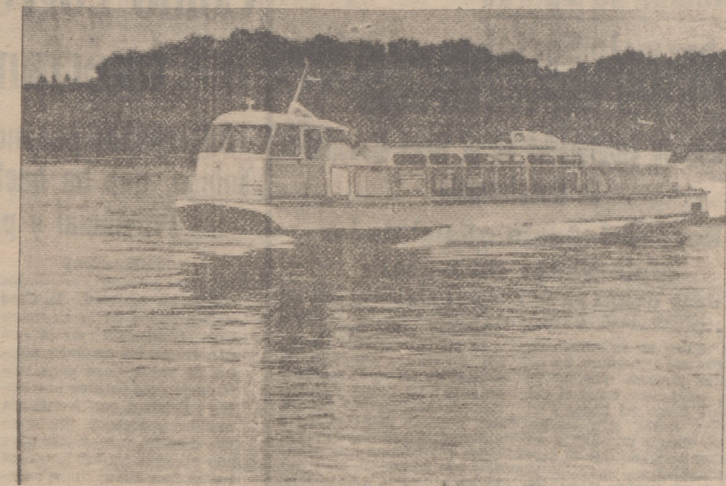
Se ha creado en la URSS un barco "semiglider", el "Opini", con motor de propulsión por agua, destinado a transporte veloz de pasajeros por ríos de poca profundidad, ya que su calado es de sólo 40 centímetros. Puede transportar a 83 pasajeros y alcanzar una velocidad de 45 kilómetros por hora. En la fotografía vemos a la embarcación durante una demostración por el río Moscova. (Foto "Fiel")
